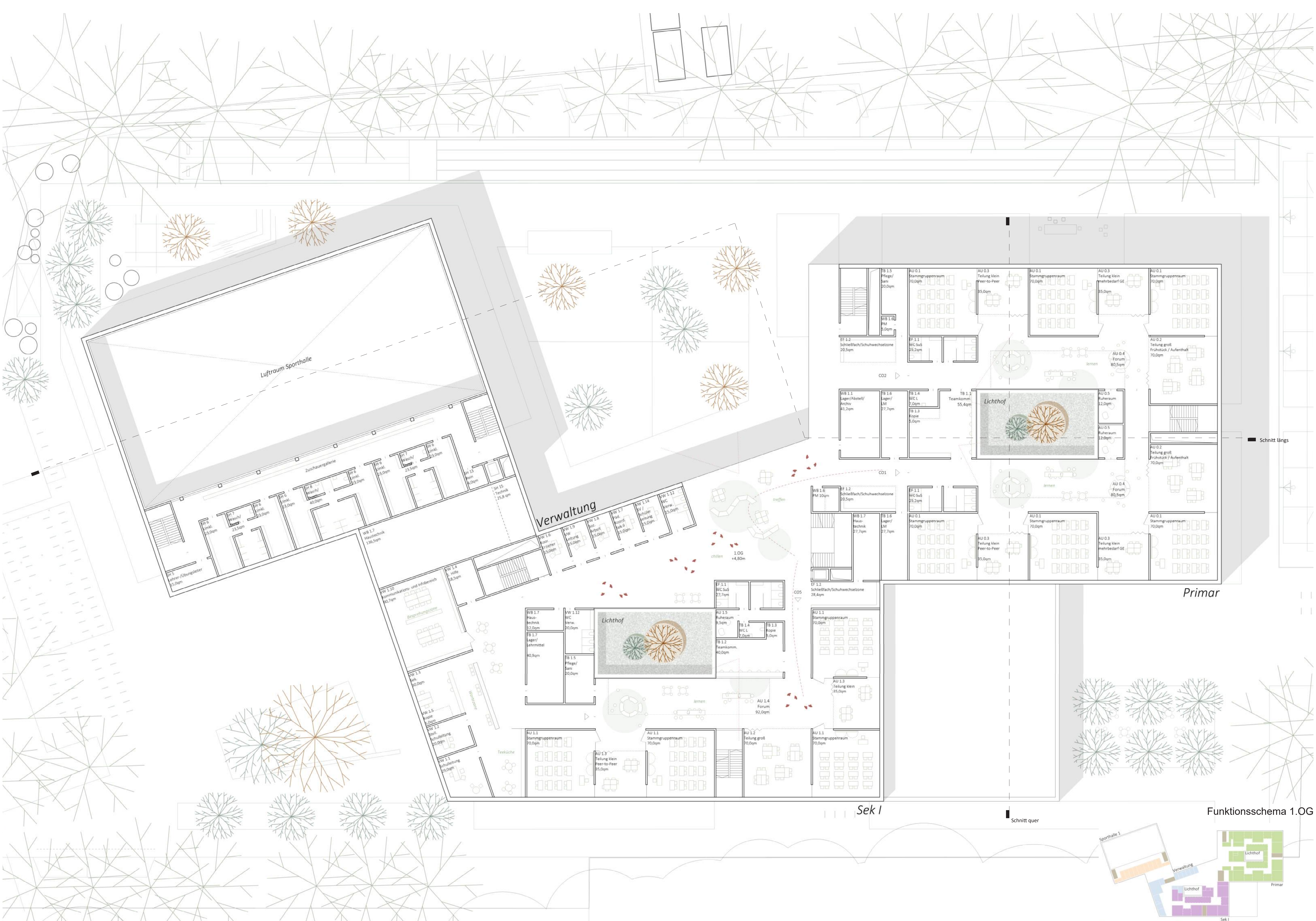
Grundriss 1. Obergeschoss 1:200
