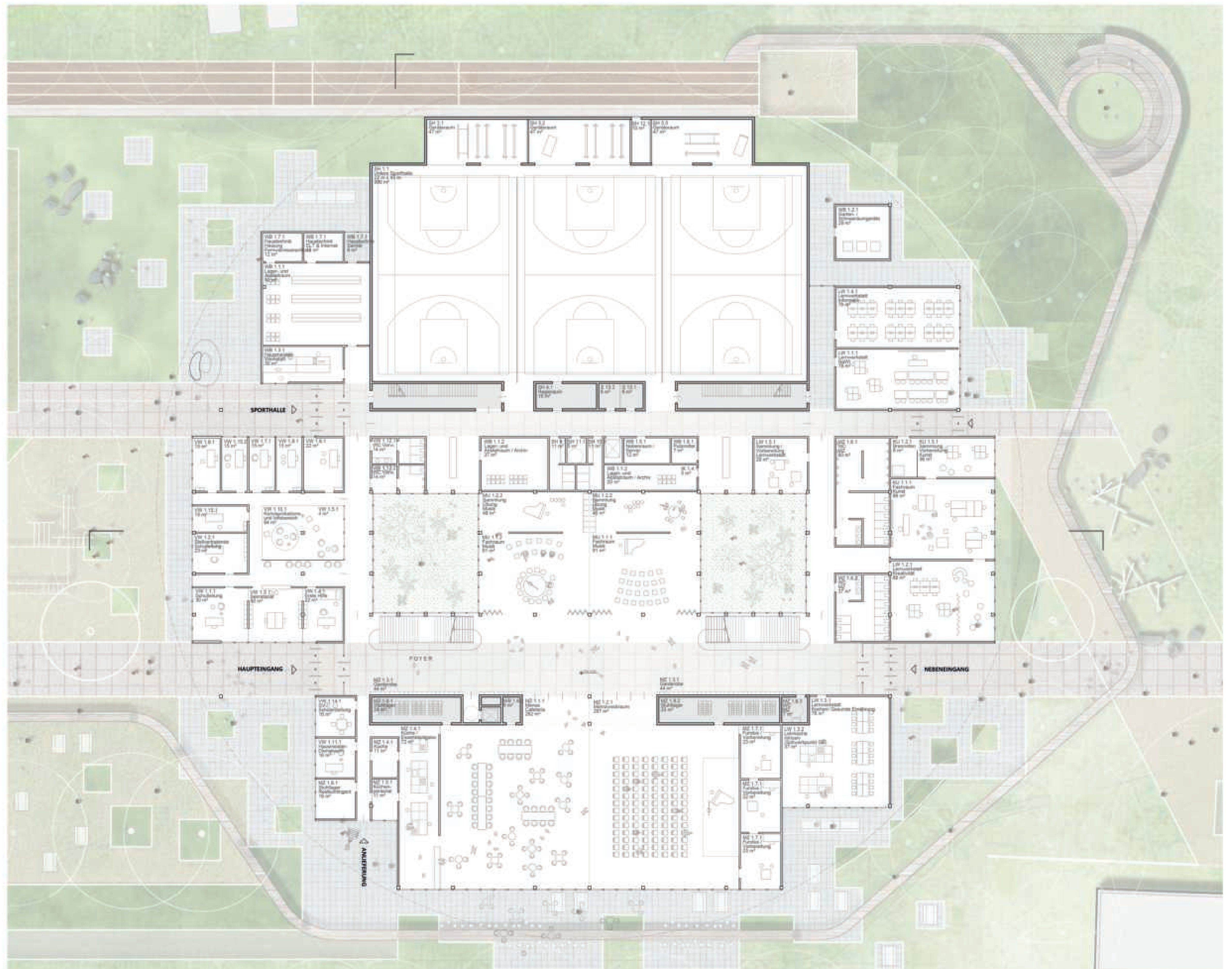
00 ERDGESCHOSS GRUNDRISS 1:200
