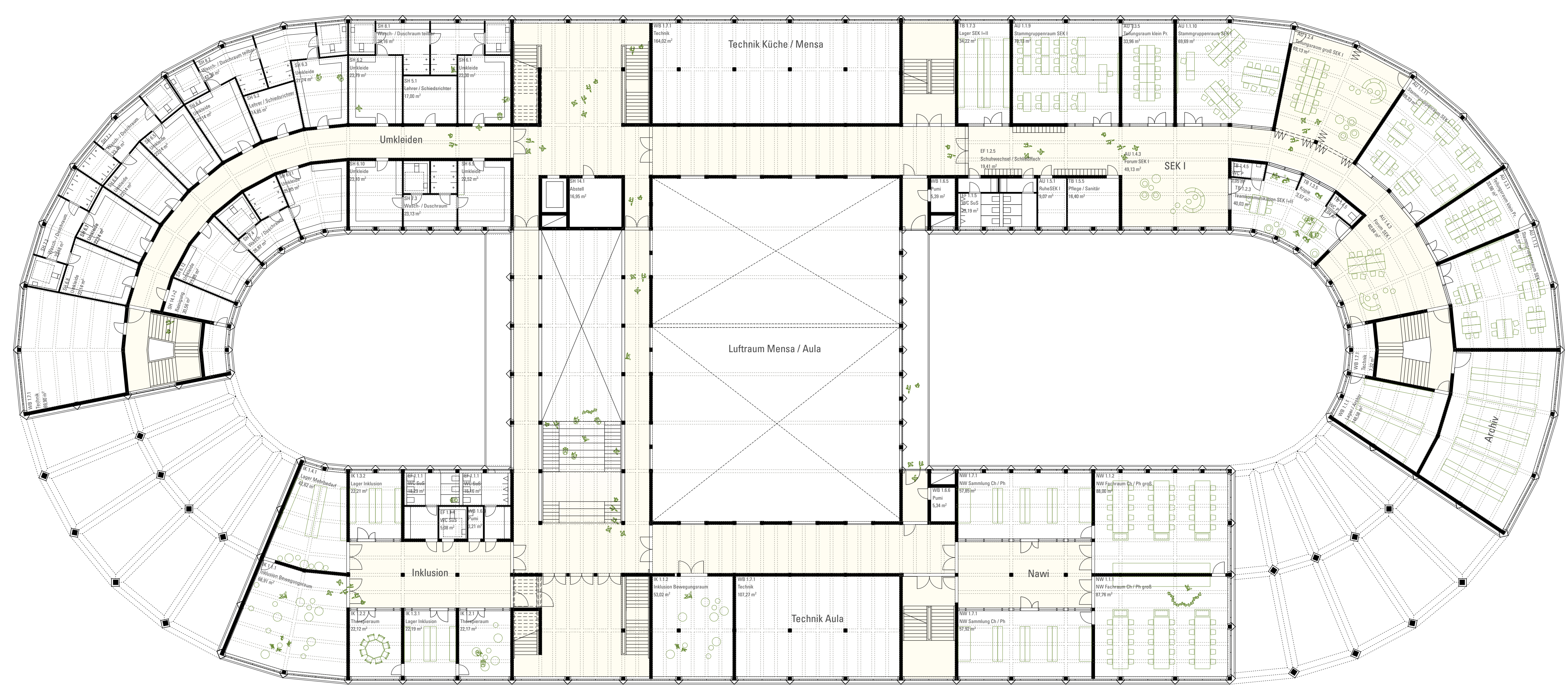
Belichtungsschema 1. OG 1:1000
