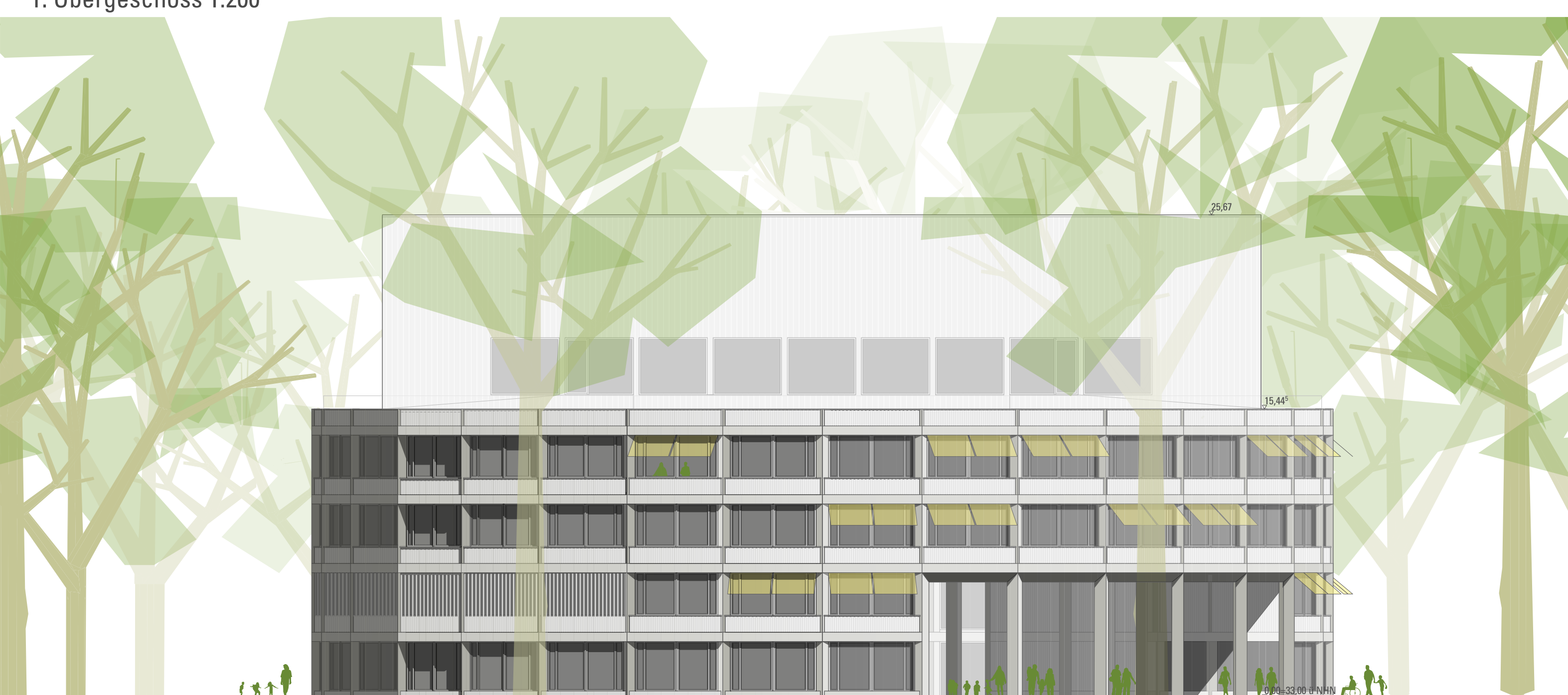
Westansicht 1:200
