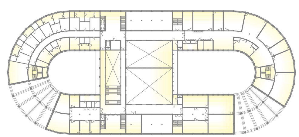
Belichtungsschema 1. OG 1:1000
