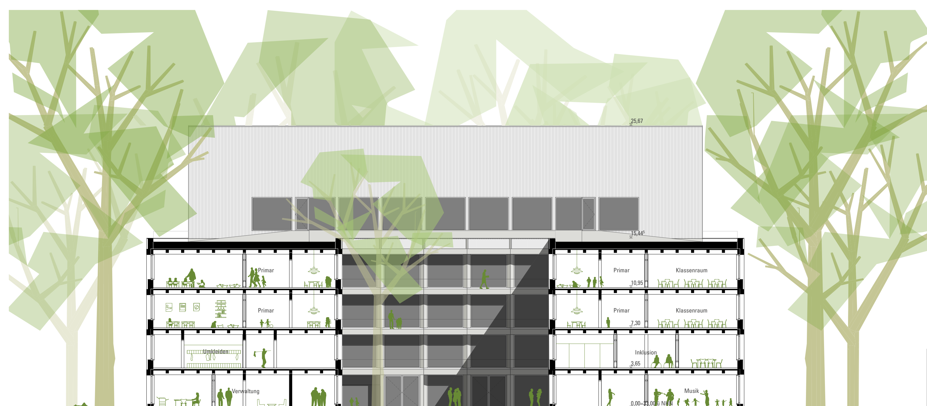
Schnitt AA 1:200
