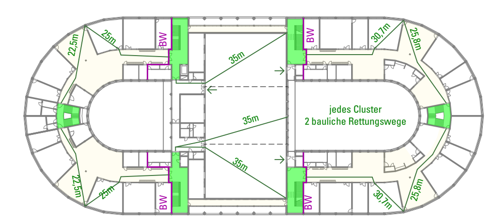
Rettungwege 2. OG 1:1000
