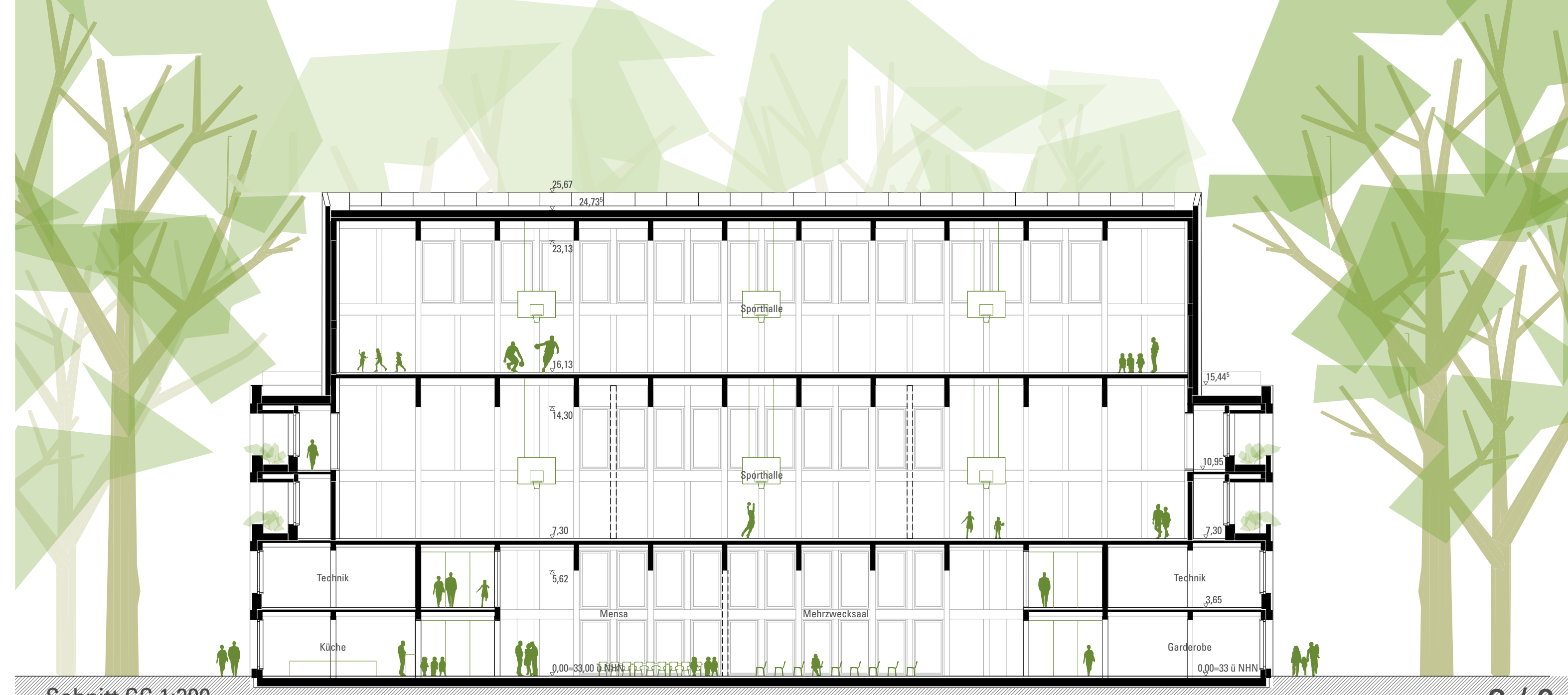
Schnitt CC 1:200
