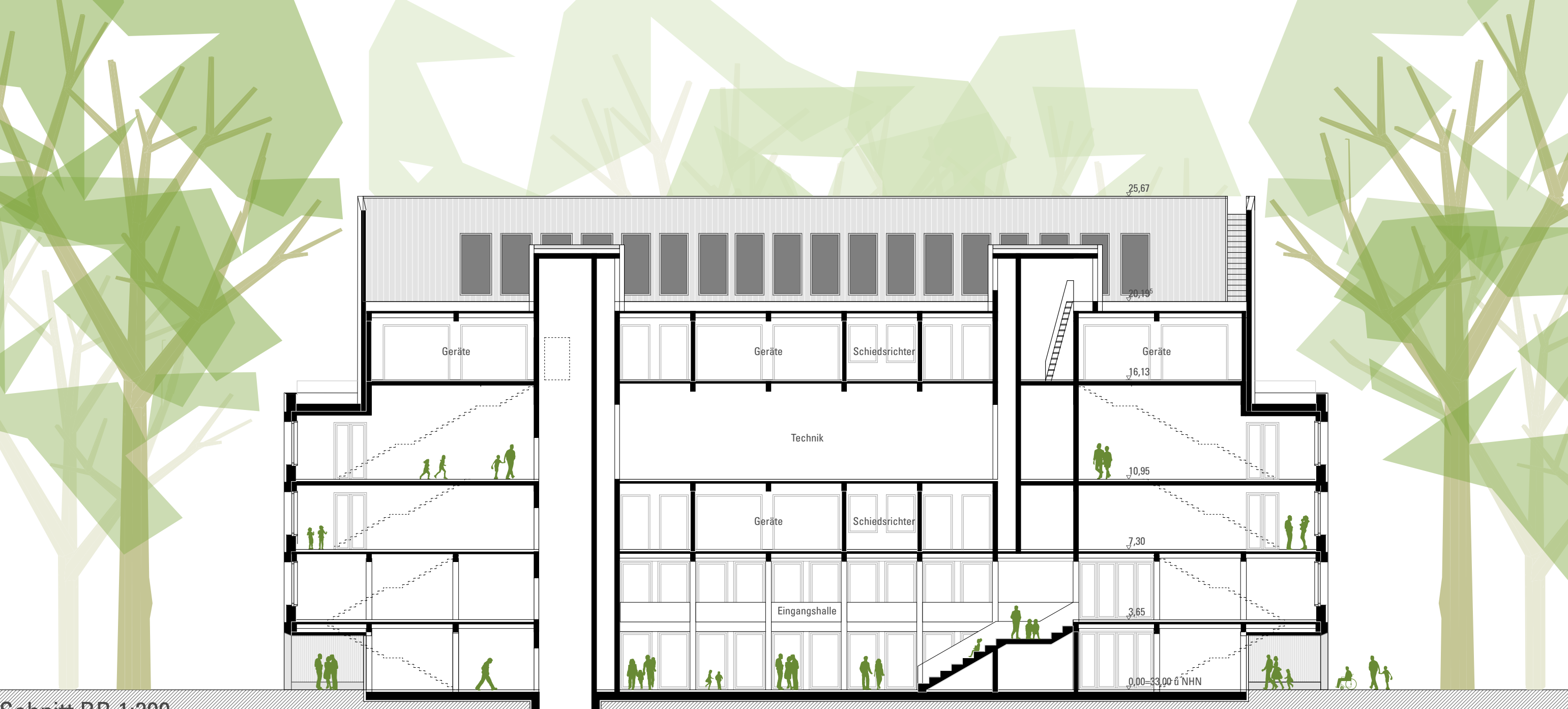
Schnitt BB 1:200
