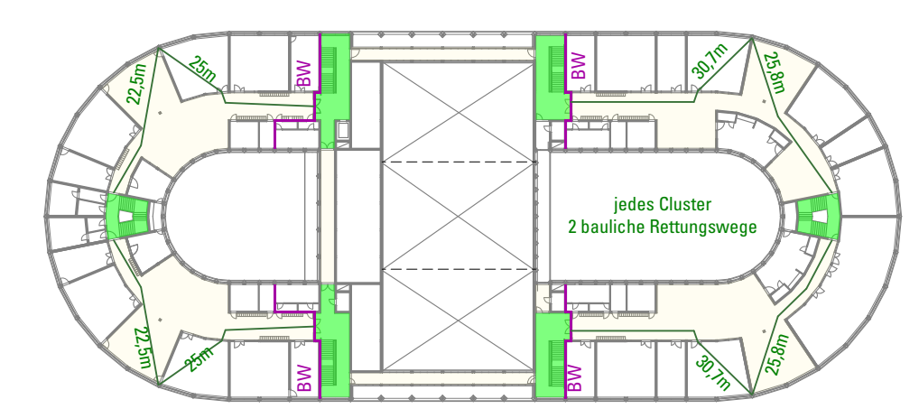
Rettungsweg 3. OG 1:1000
