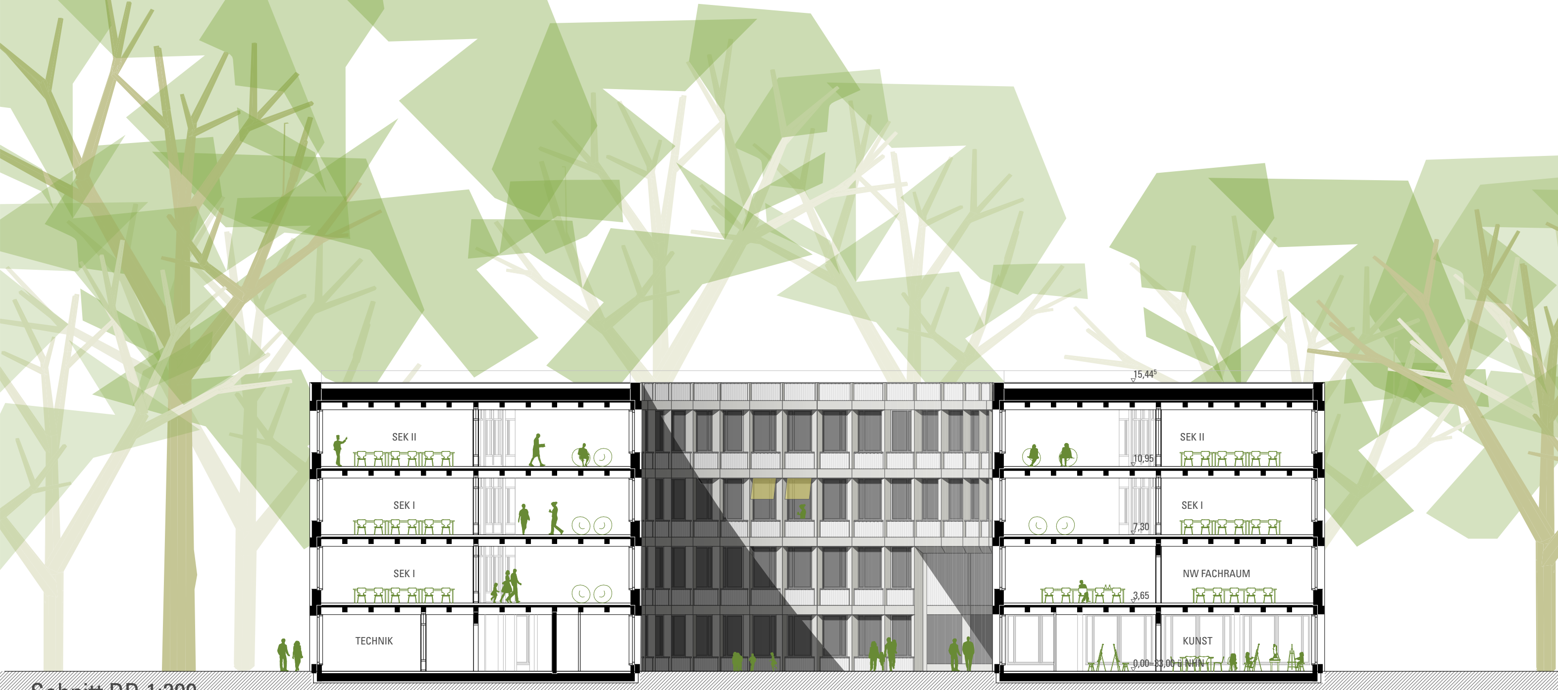
Schnitt DD 1:200
