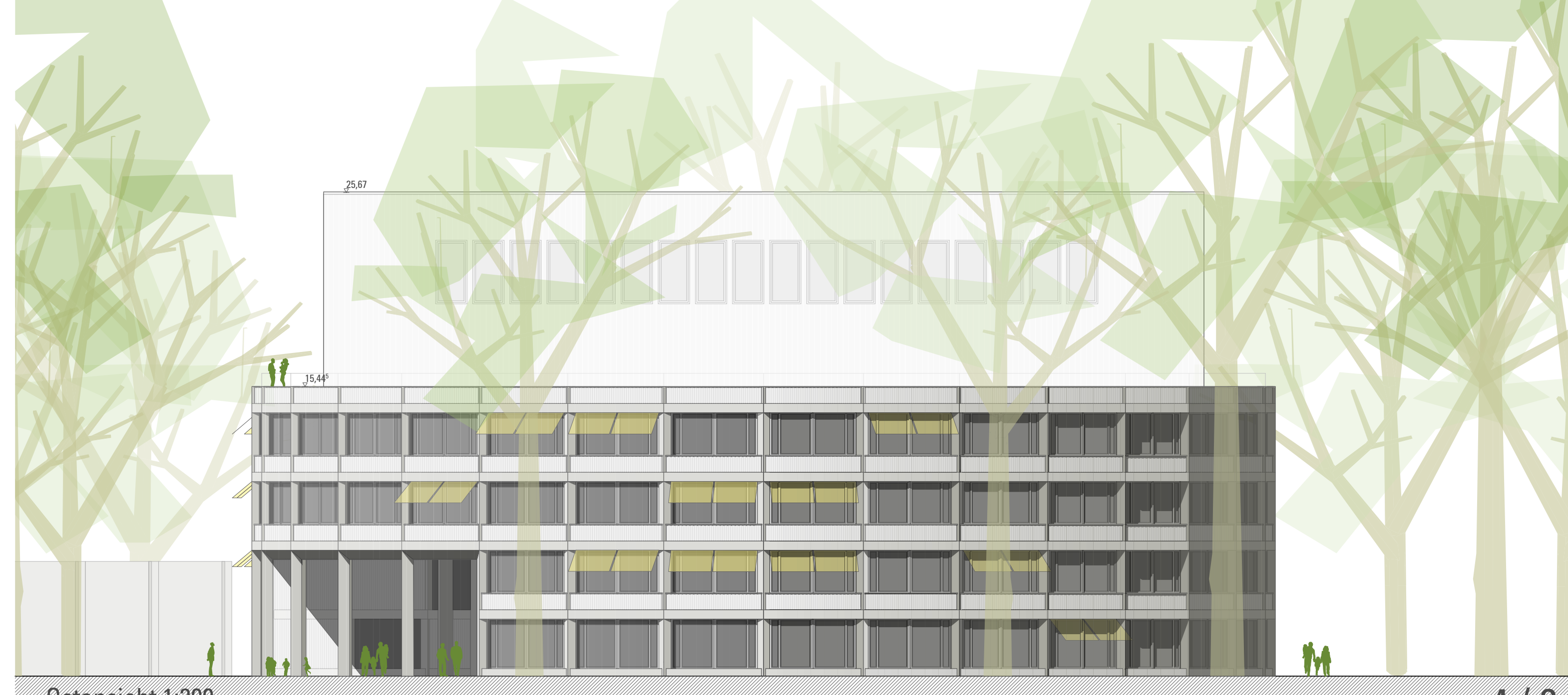
Ostansicht 1:200
