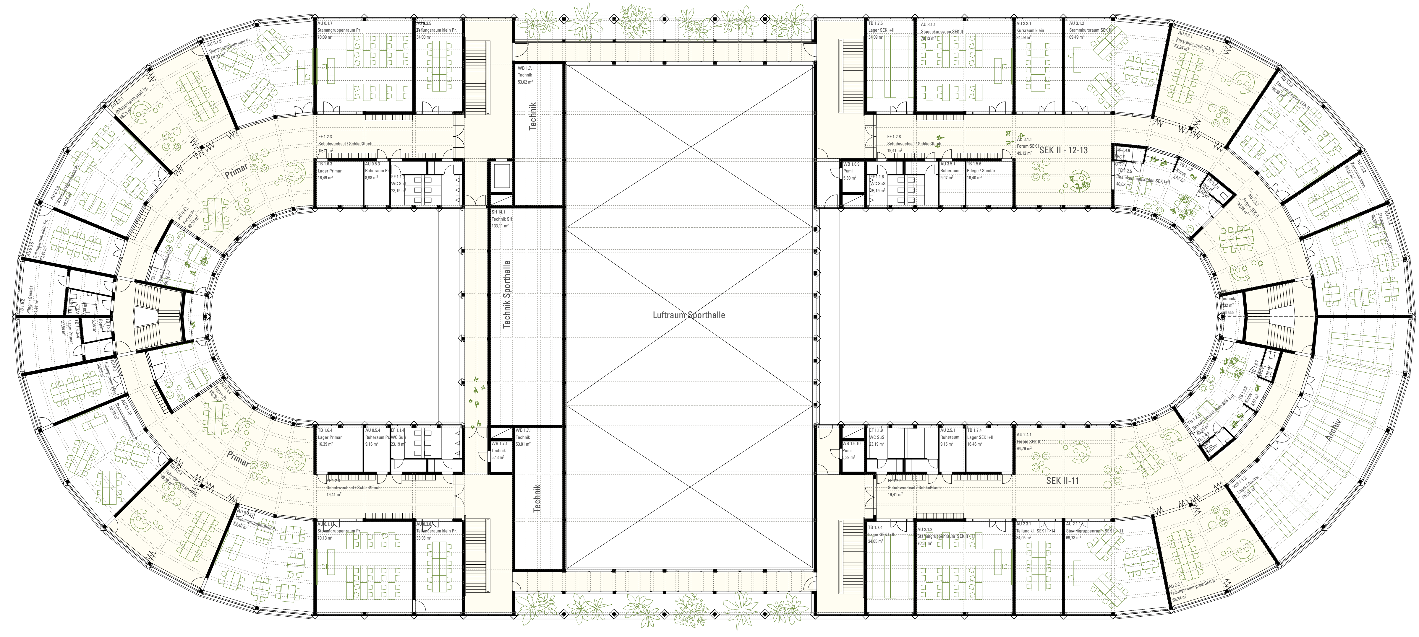
Belichtungsschema 3. OG 1:1000
