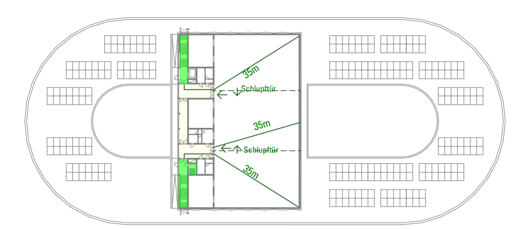
Rettungswege DG 1:1000
