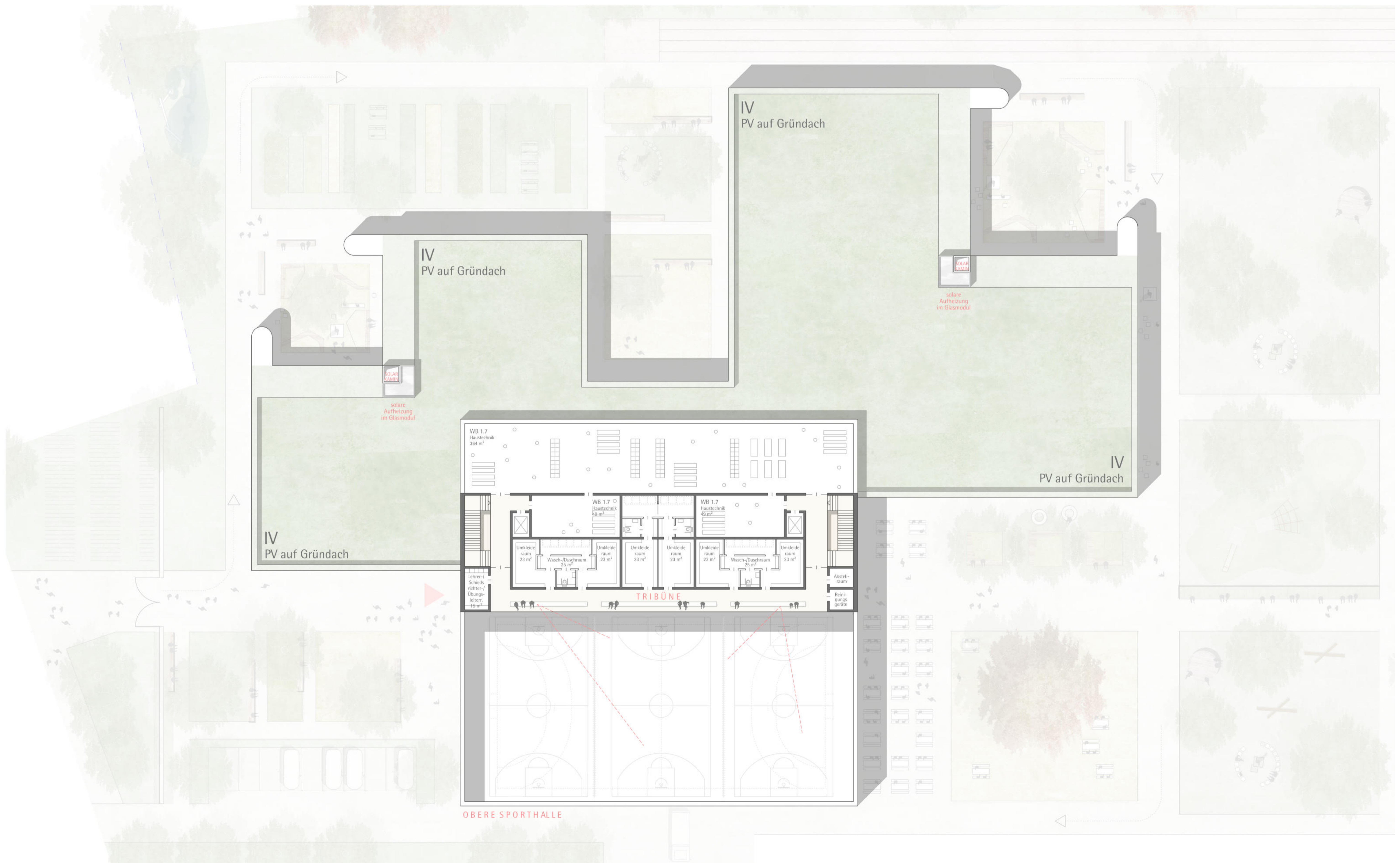
GRUNDRISS 4.OBERGESCHOSS M 1:200
