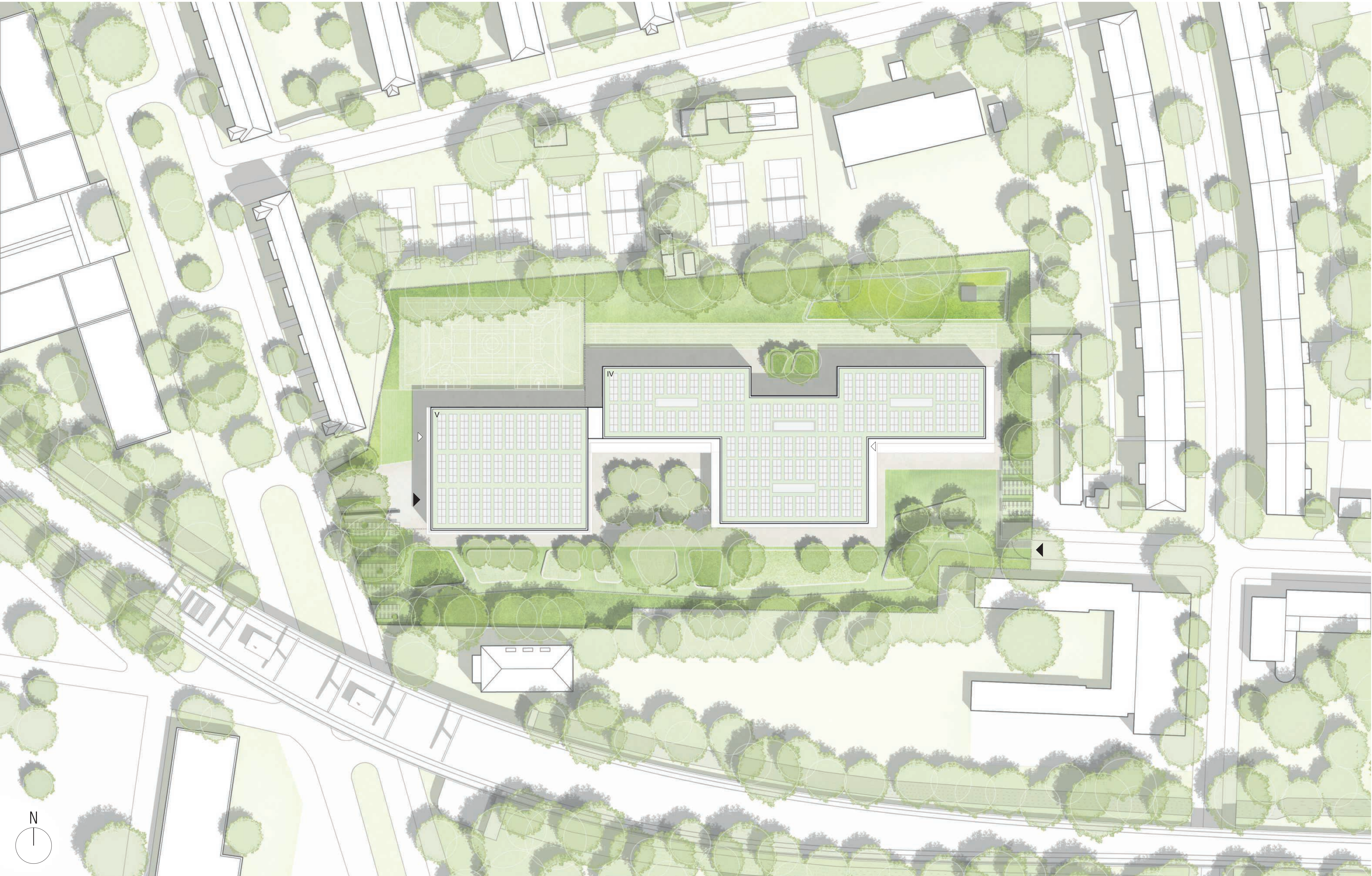
LAGEPLAN M 1:500
