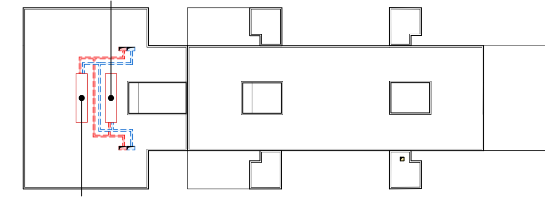
Schema TGA Dach M 1:1000
