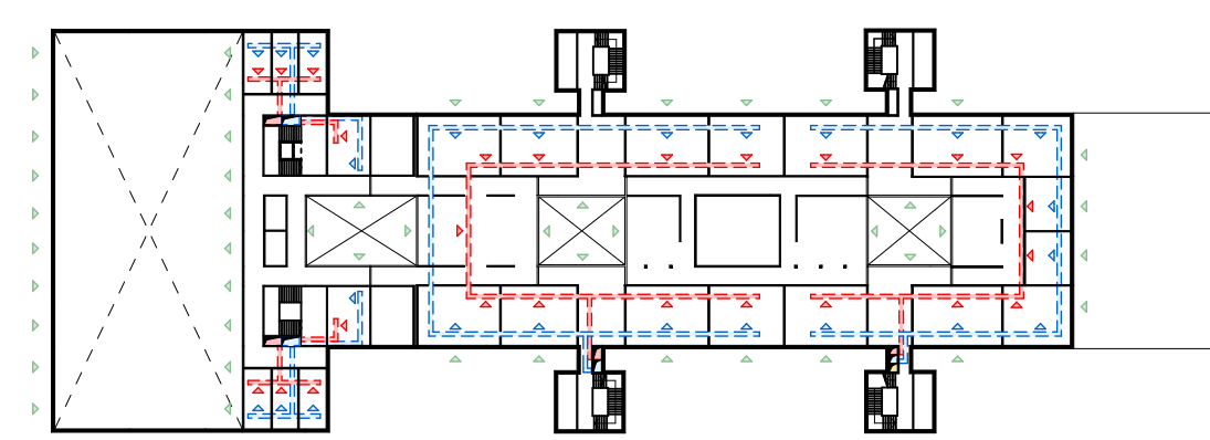
Schema TGA 3. Obergeschoss M 1:1000
