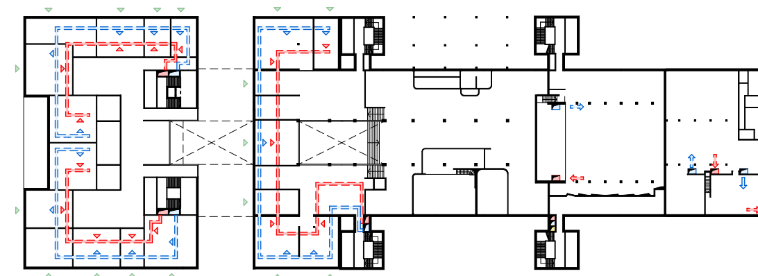
Schema TGA Erdgeschoss M 1:1000
