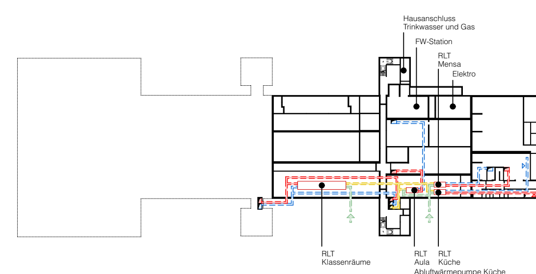
Schema TGA Untergeschoss M 1:1000
