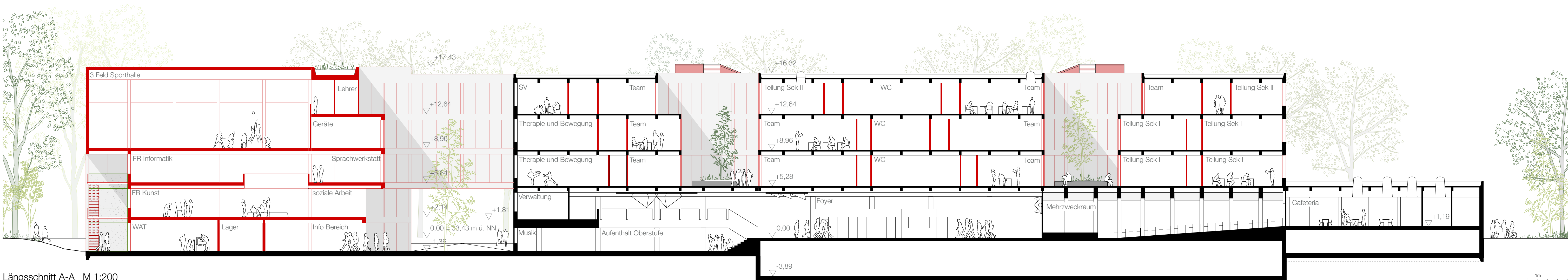
Längsschnitt A-A M 1:200
