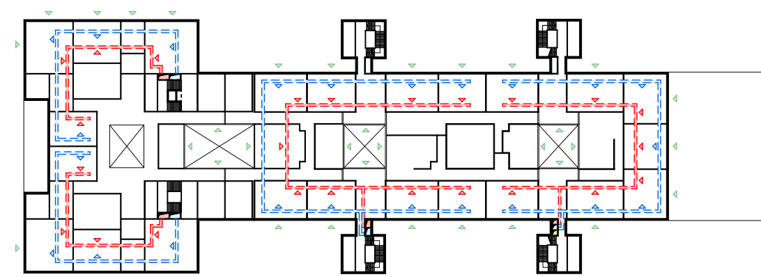
Schema TGA 1. Obergeschoss M 1:1000
