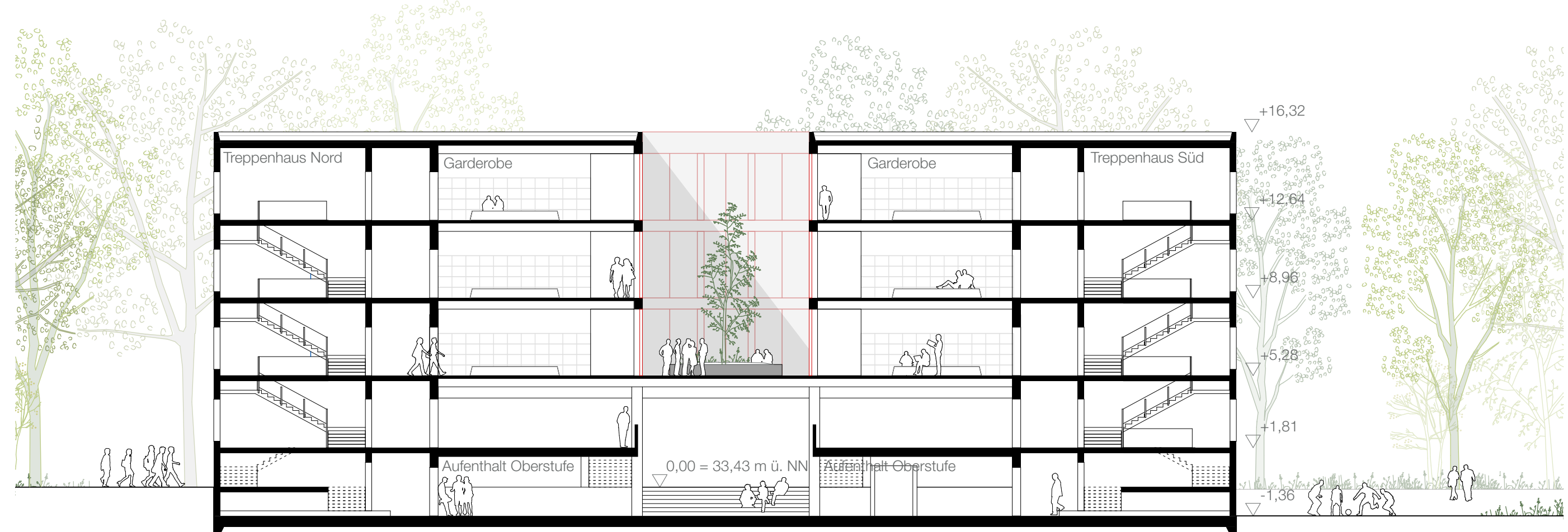
Querschnitt D-D M 1:200
