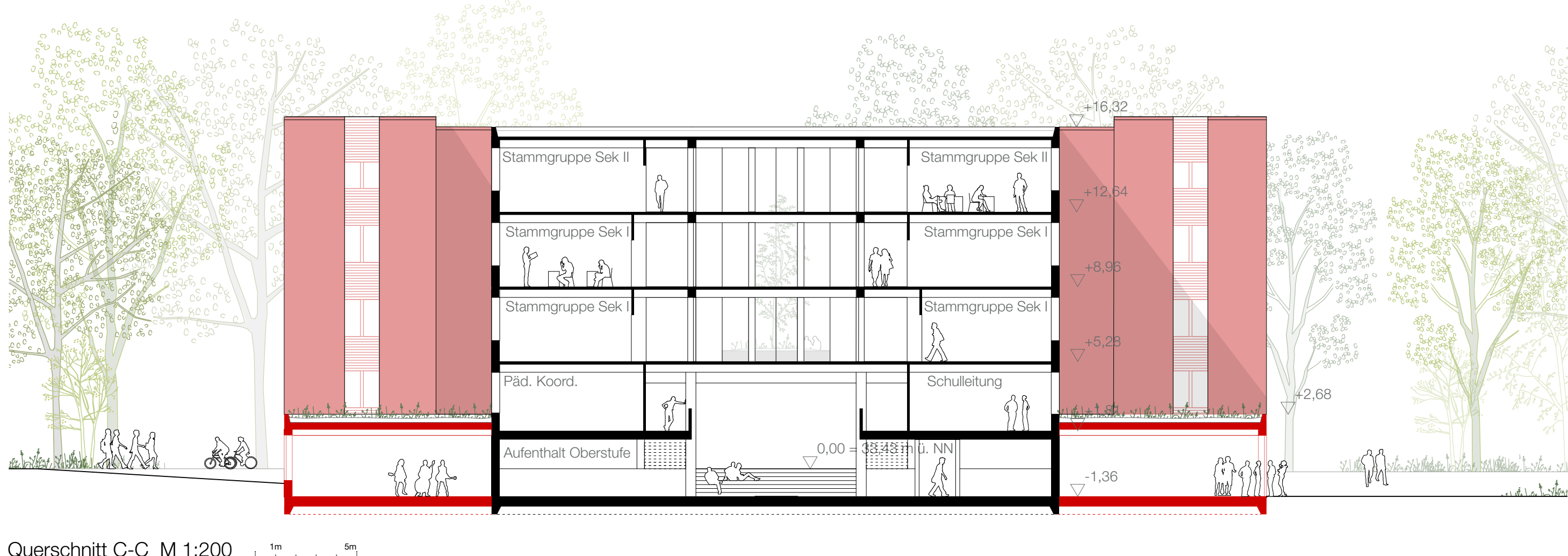
Querschnitt C-C M 1:200
