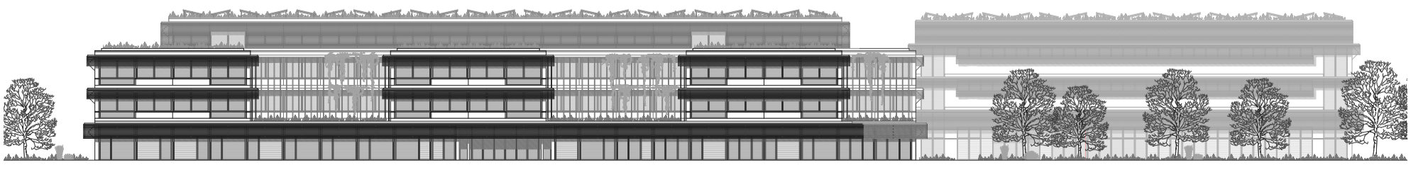
Ansicht Süd
