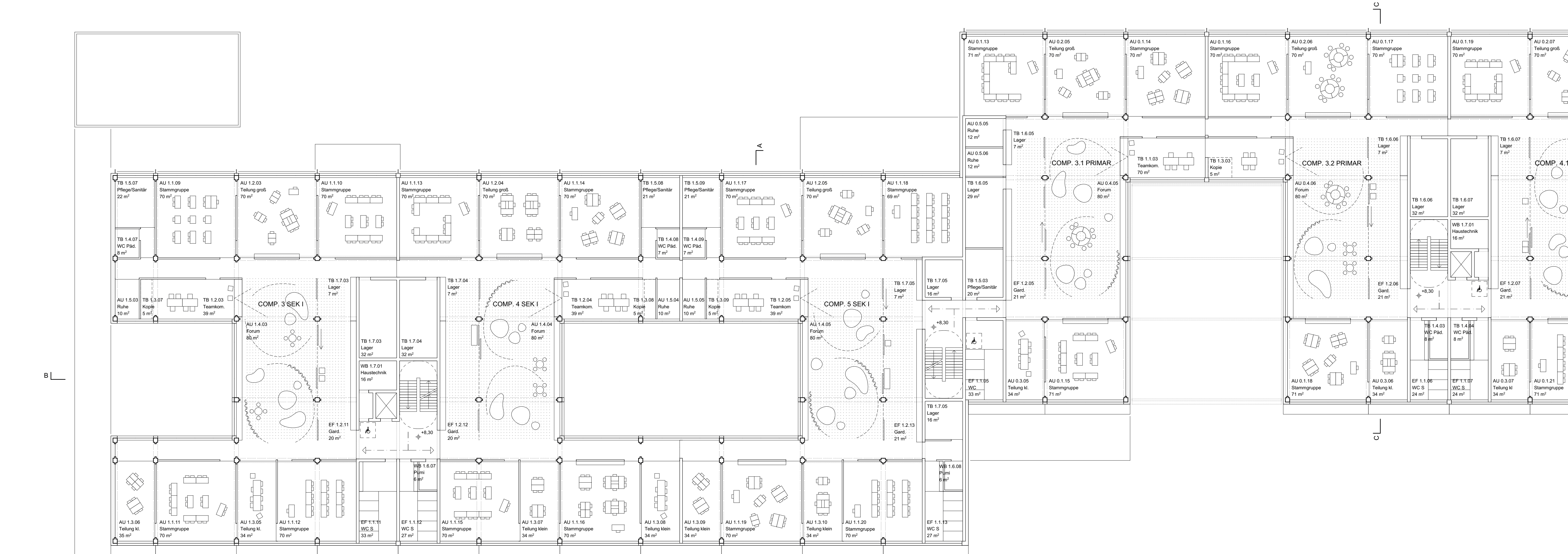
GRUNDRISS 2. OBERGESCHOSS M 1:200
