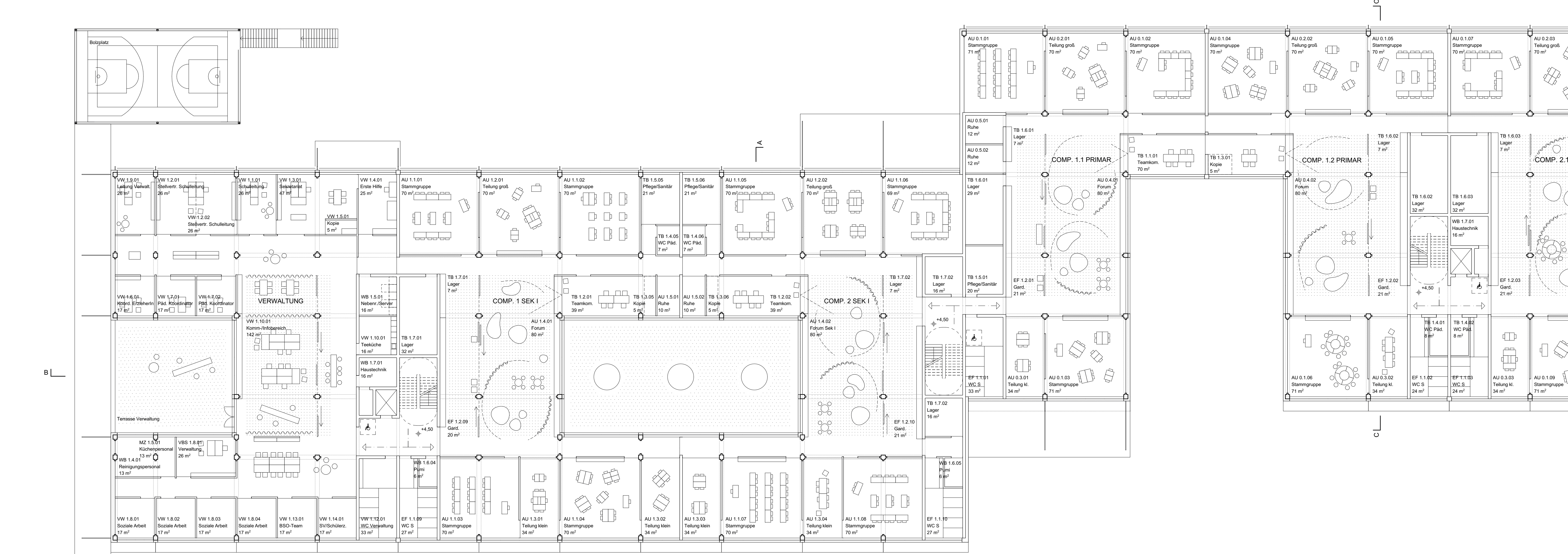
GRUNDRISS 1. OBERGESCHOSS M 1:200
