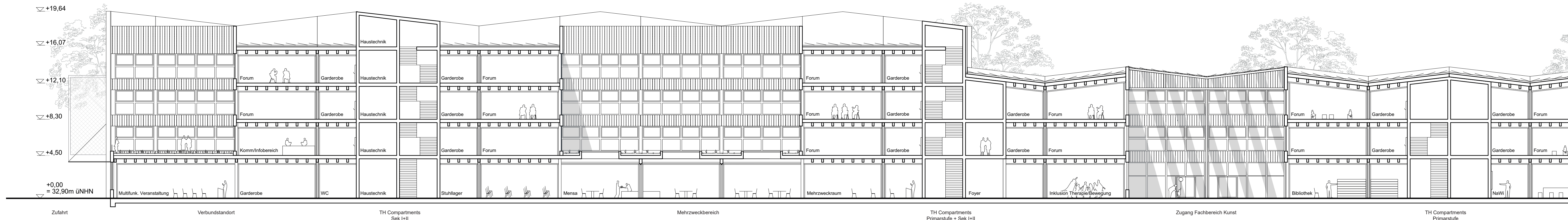
LÄNGSSCHNITT B M 1:200
