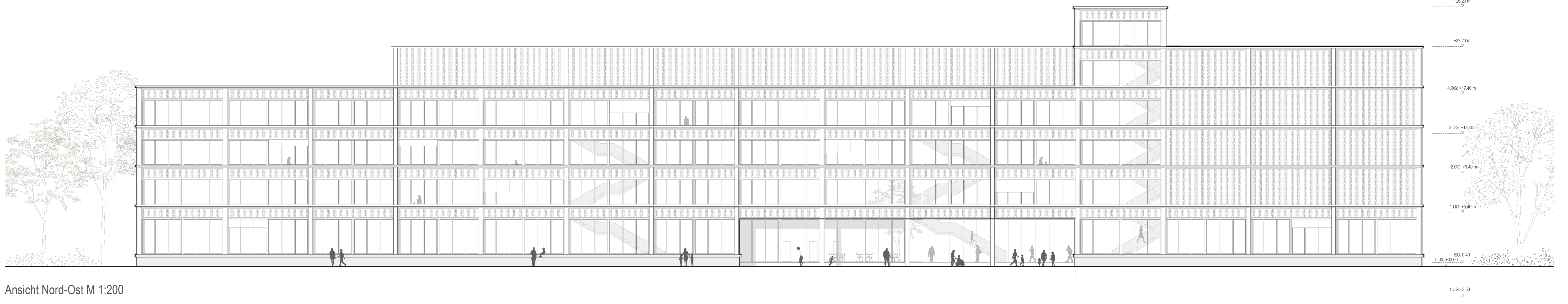
Ansicht Nord-Ost M 1:200
