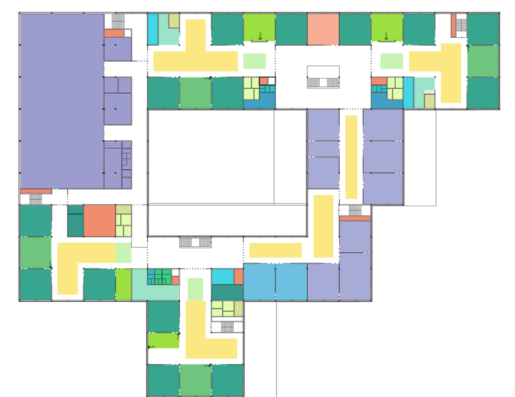
Funktionsdiagramm 3.OG M 1:1000
