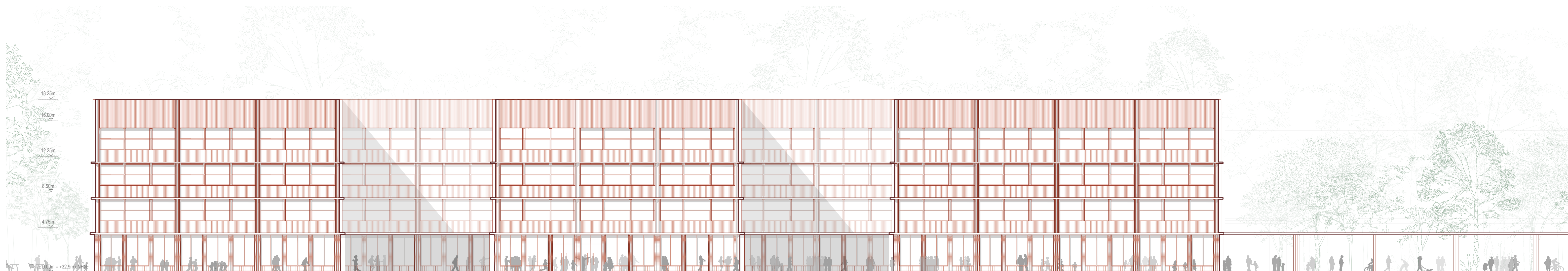
ANSICHT NORD 1:200
