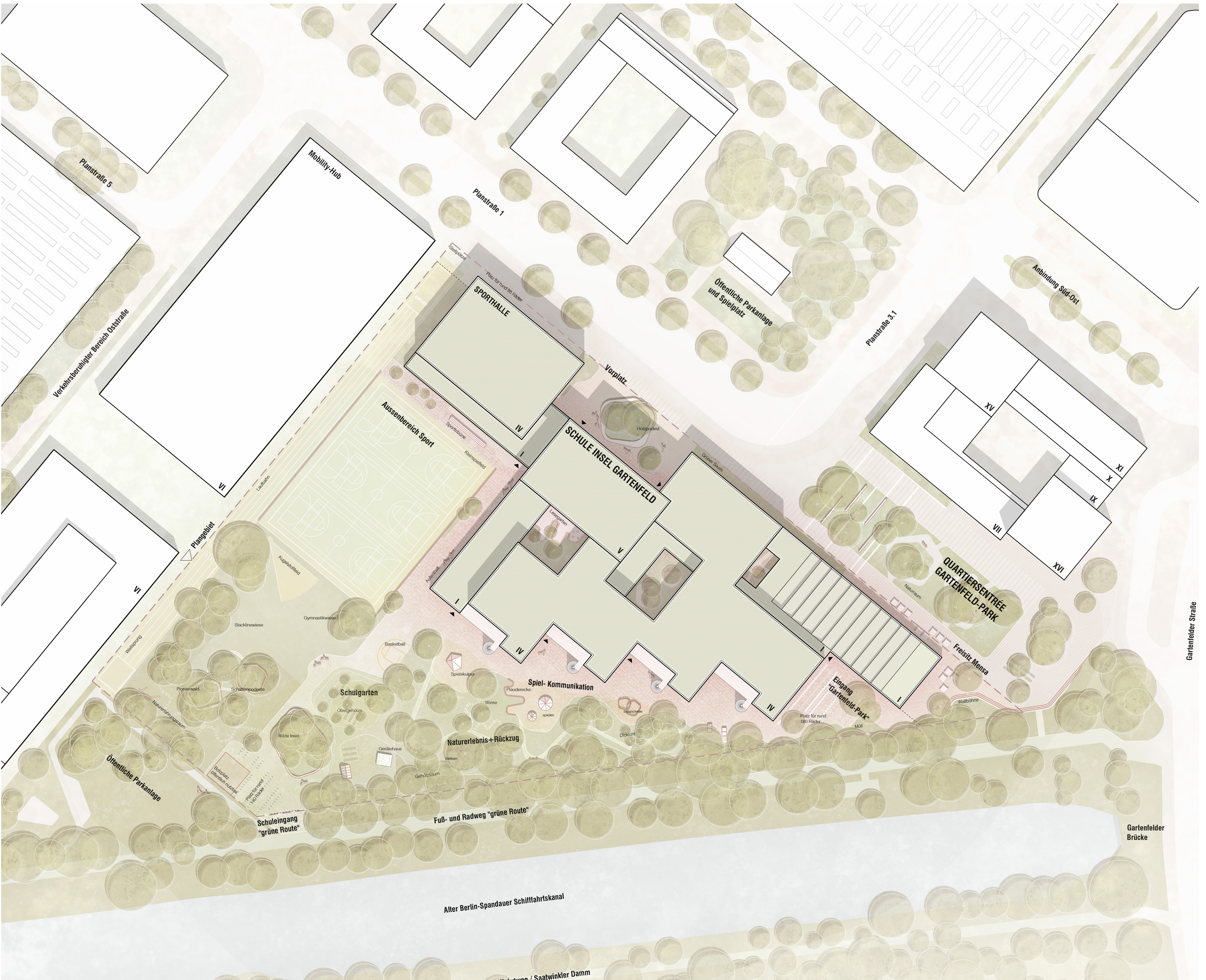
LAGEPLAN
