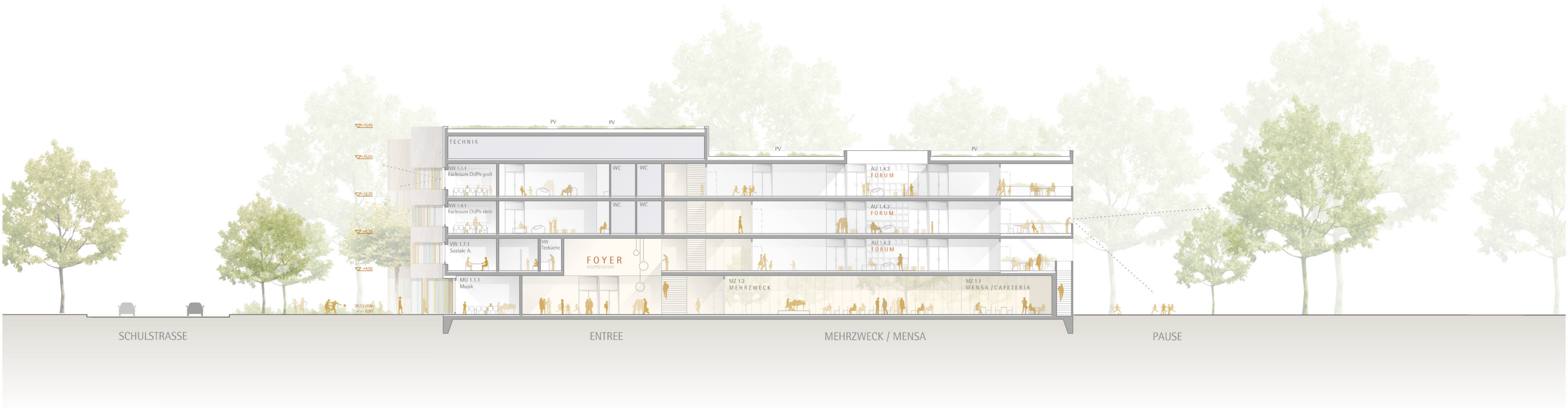
SCHNITT A-A M 1:200
