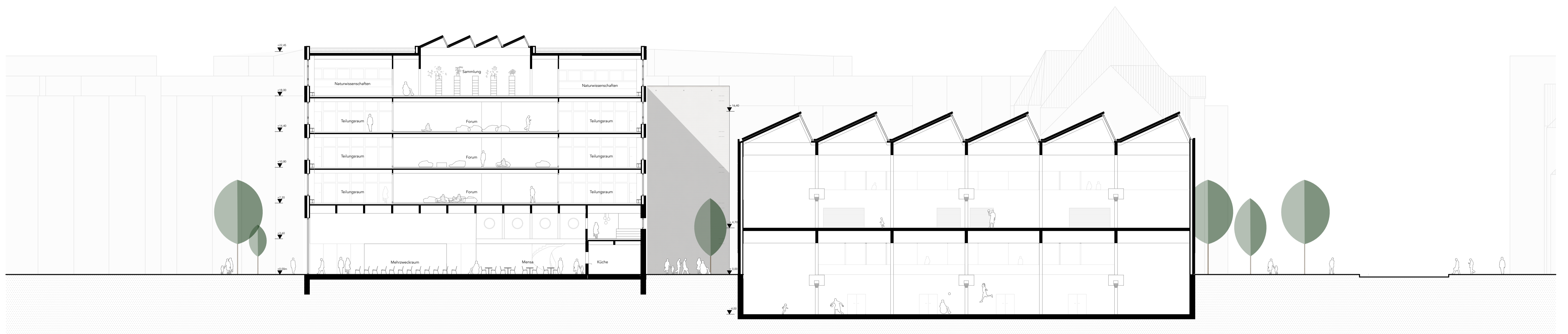
SCHNITT B-B SCHULE UND HALLE M.1:200
