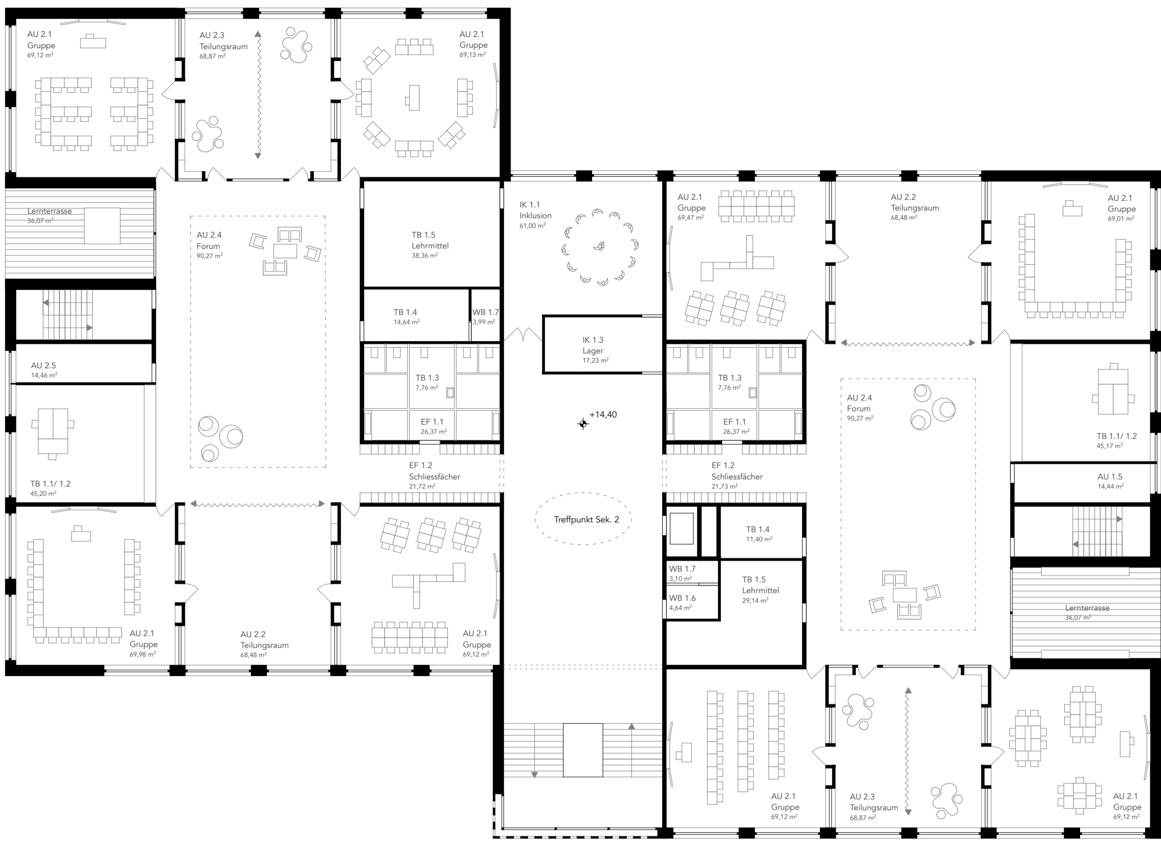
GRUNDRISS 3. OBERGESCHOSS SCHULE M.1:200
