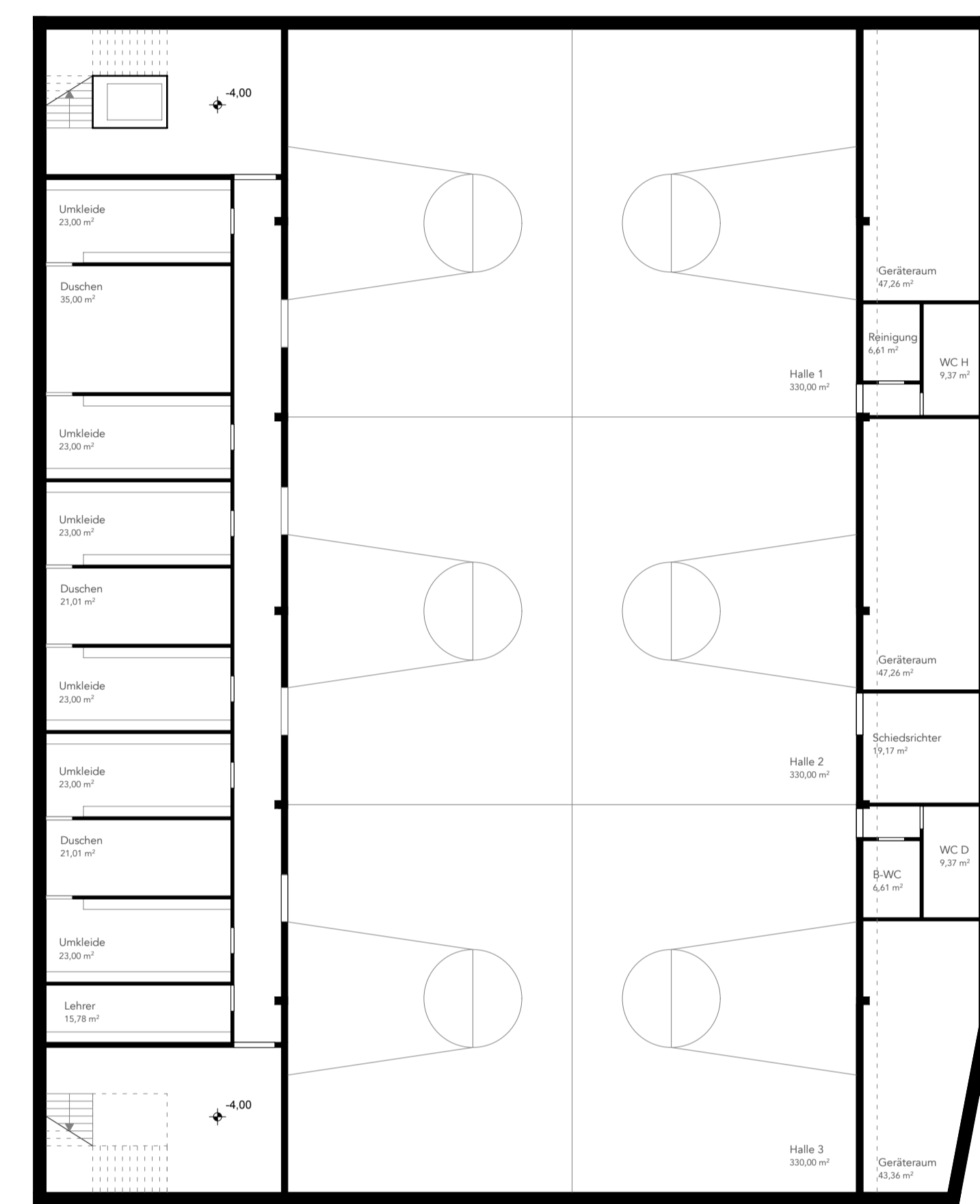
GRUNDRISS UNTERGESCHOSS HALLE M.1:200
