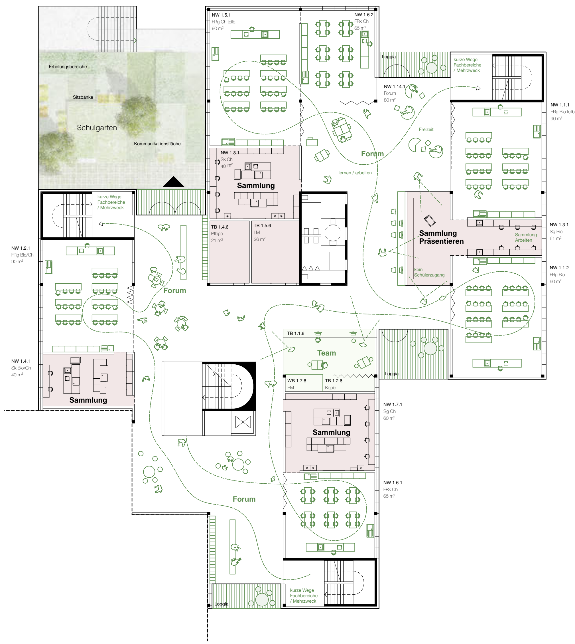
Möbelierung Fachraum Compartment Biologie/Chemie 1.OG M 1:200
