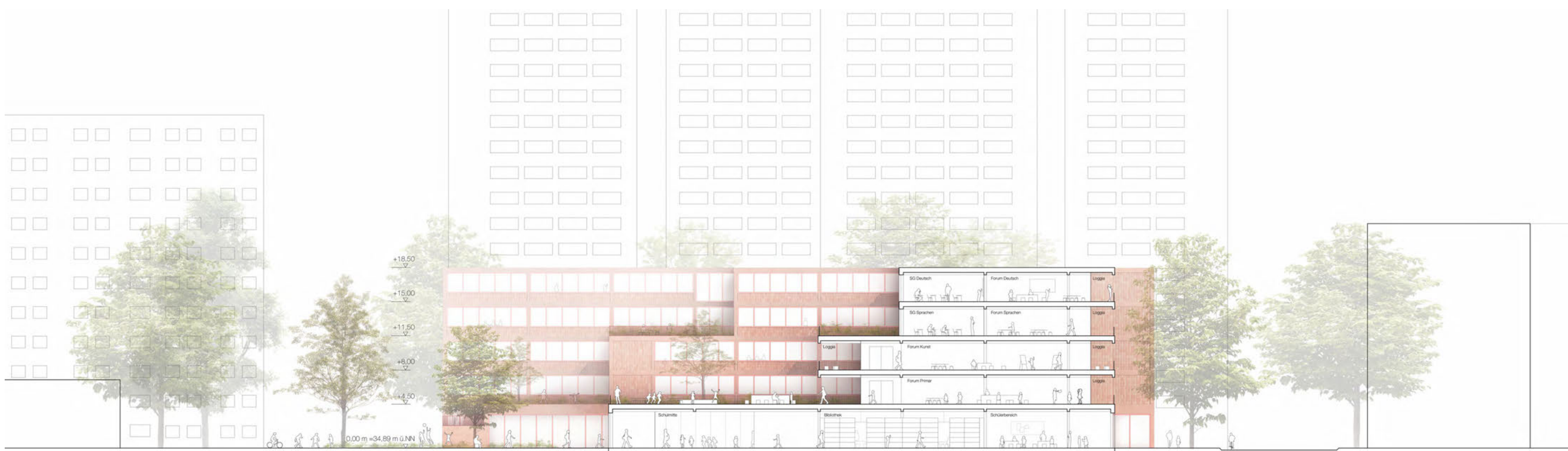
Schnitt S2/ Ansicht West M 1:200
