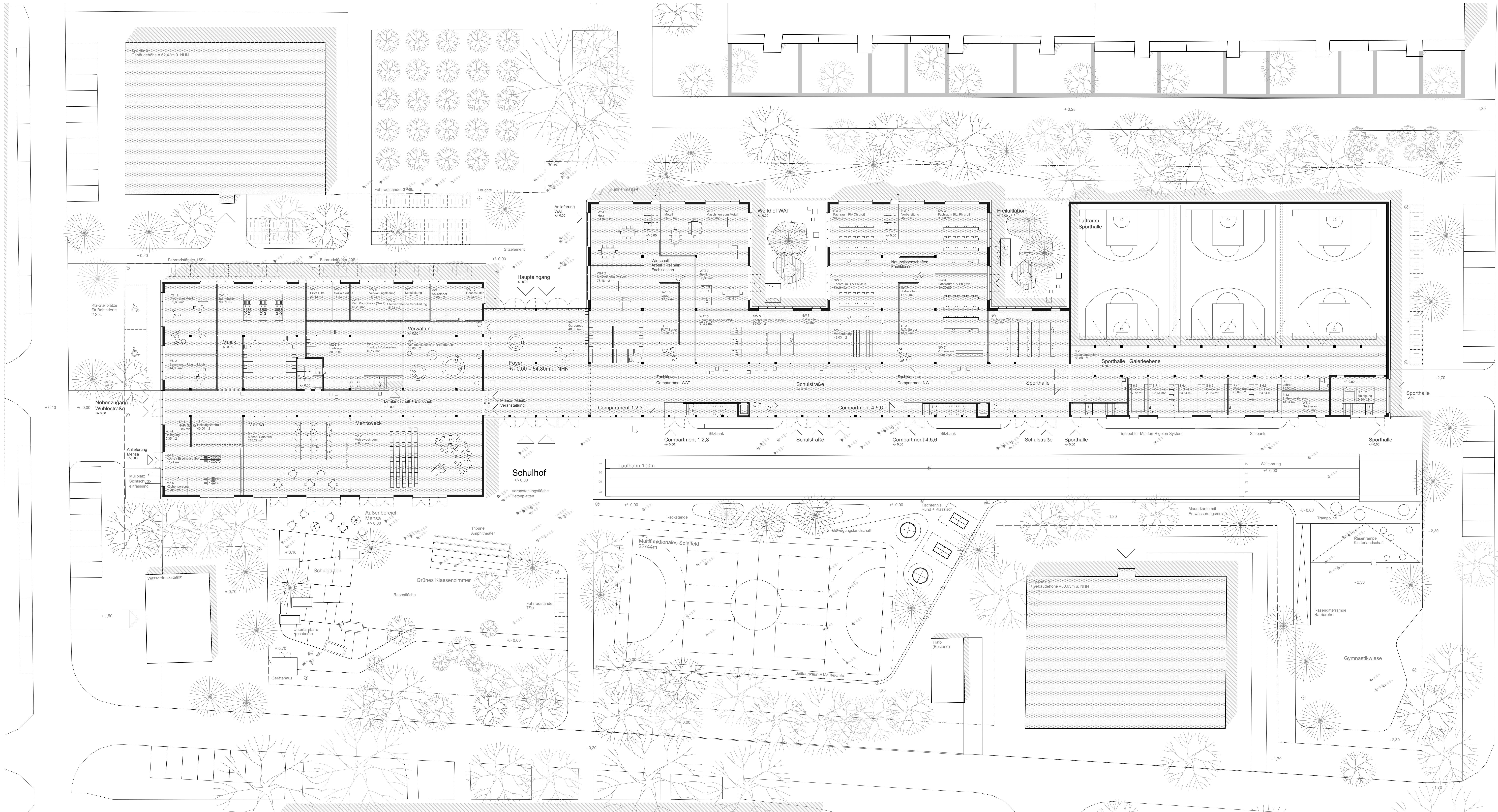
Grundriss Erdgeschoss/ Galerieebene Sporthalle M 1:200
