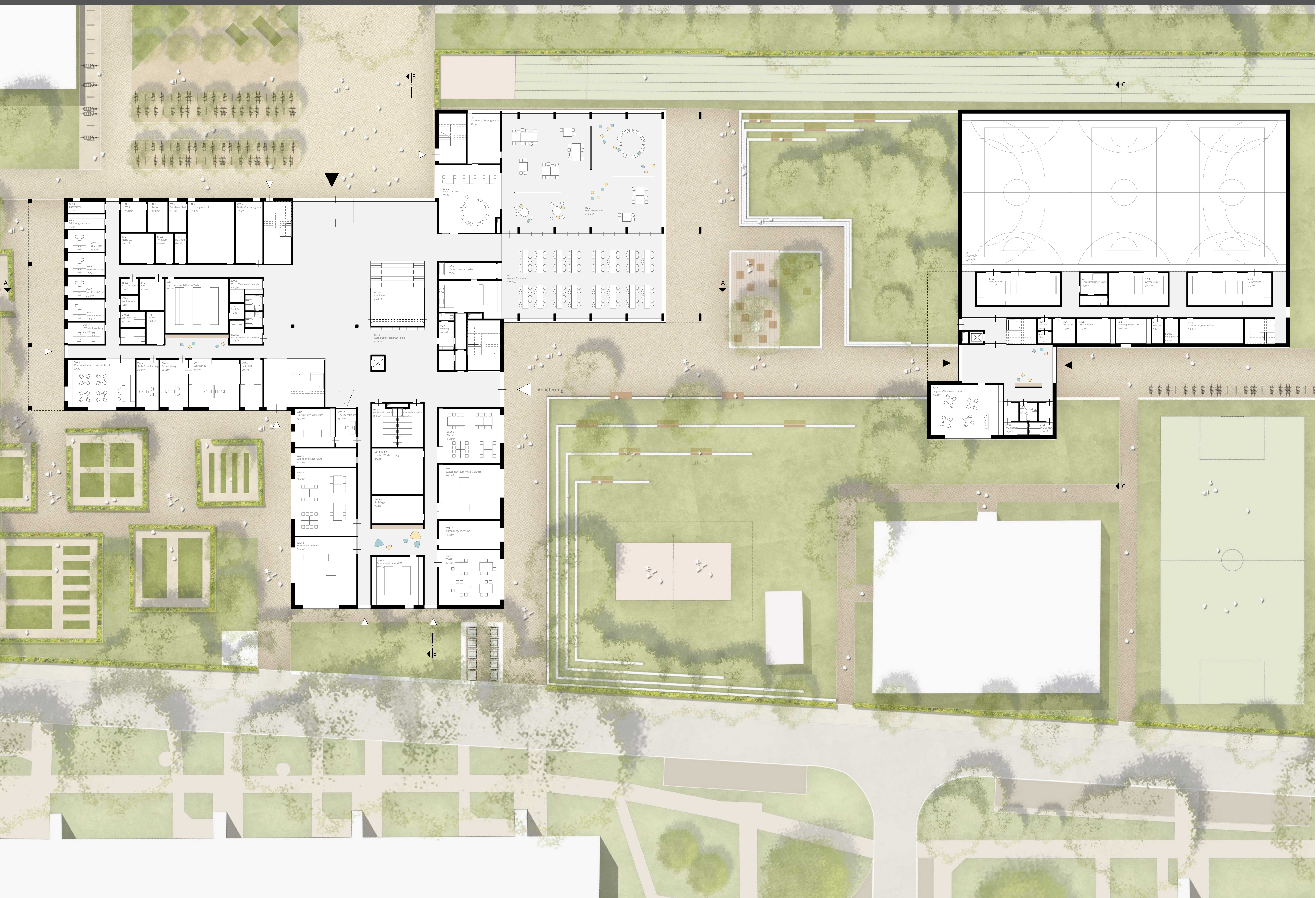
GRUNDRISS EG | 1:200
