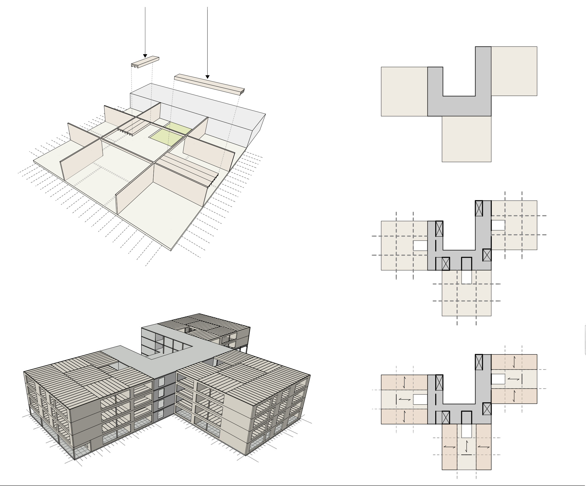
SCHEMA | MODULBAUWEISE
