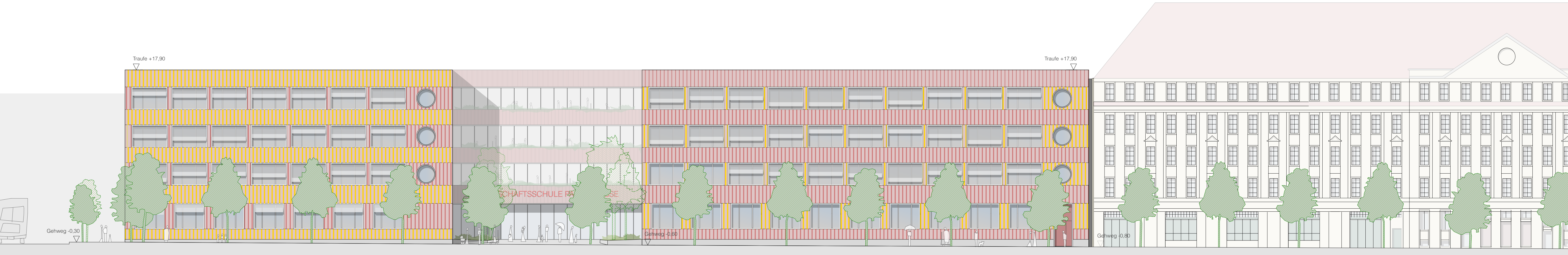
Ansicht Schönstedtstrasse M 1:200
