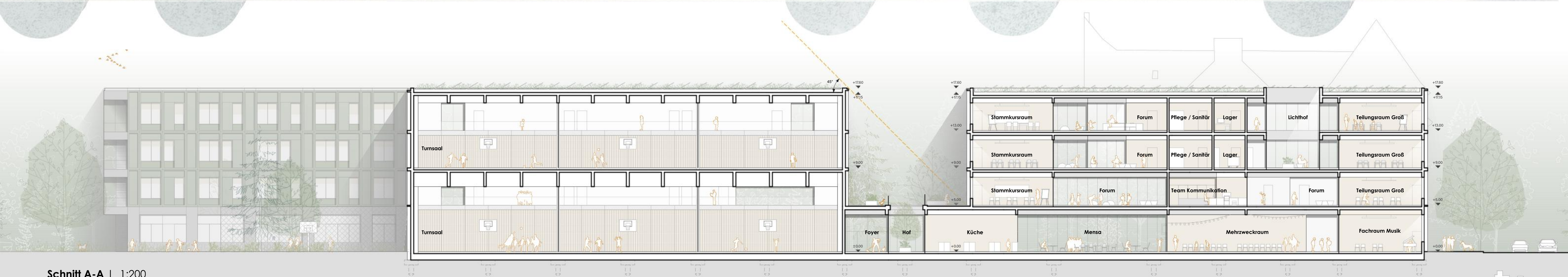
Schnitt A-A | 1:200
