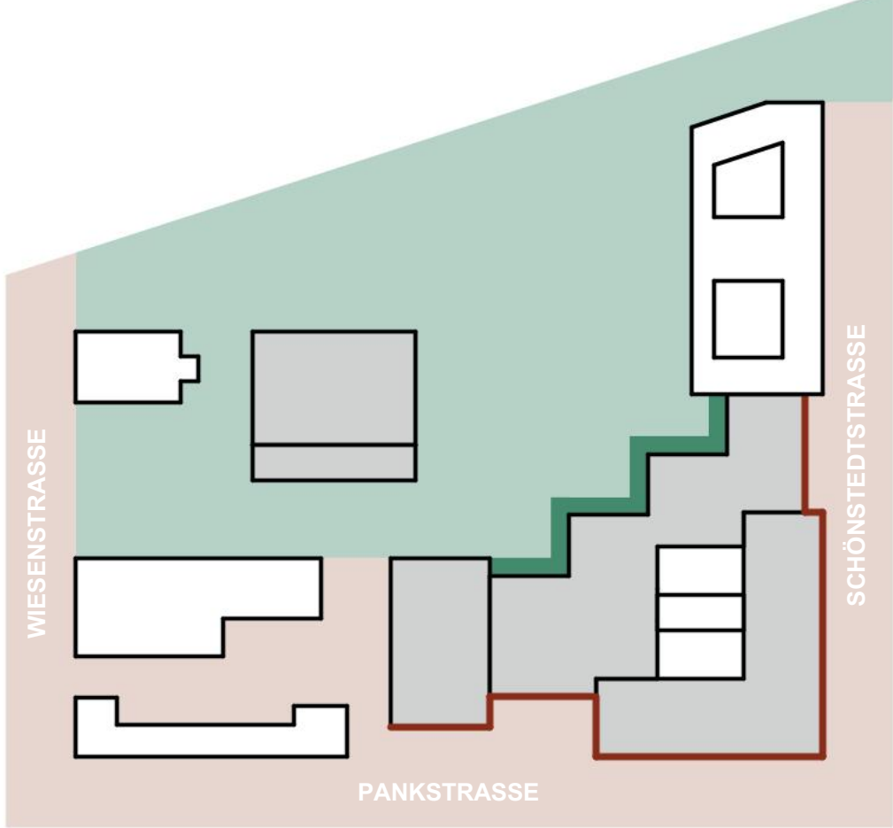
STADT- UND FREIRAUM Die neue Schule ergänzt die räumliche Fassung des Brunnenplatzes. Zum Pausenhof verzahnt sich der Baukörper mit dem durchgrüntem Freiraum.
