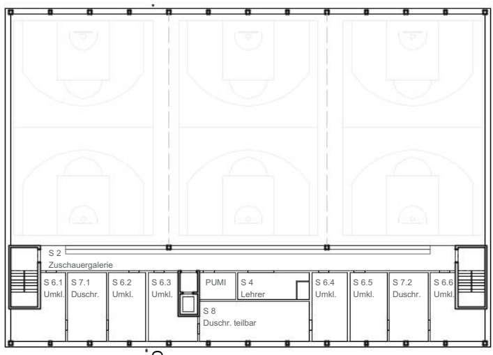
Sporthalle 3. OG 1:500
