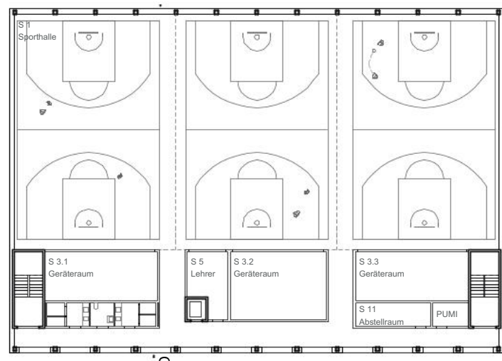
Sporthalle 2. OG 1:500
