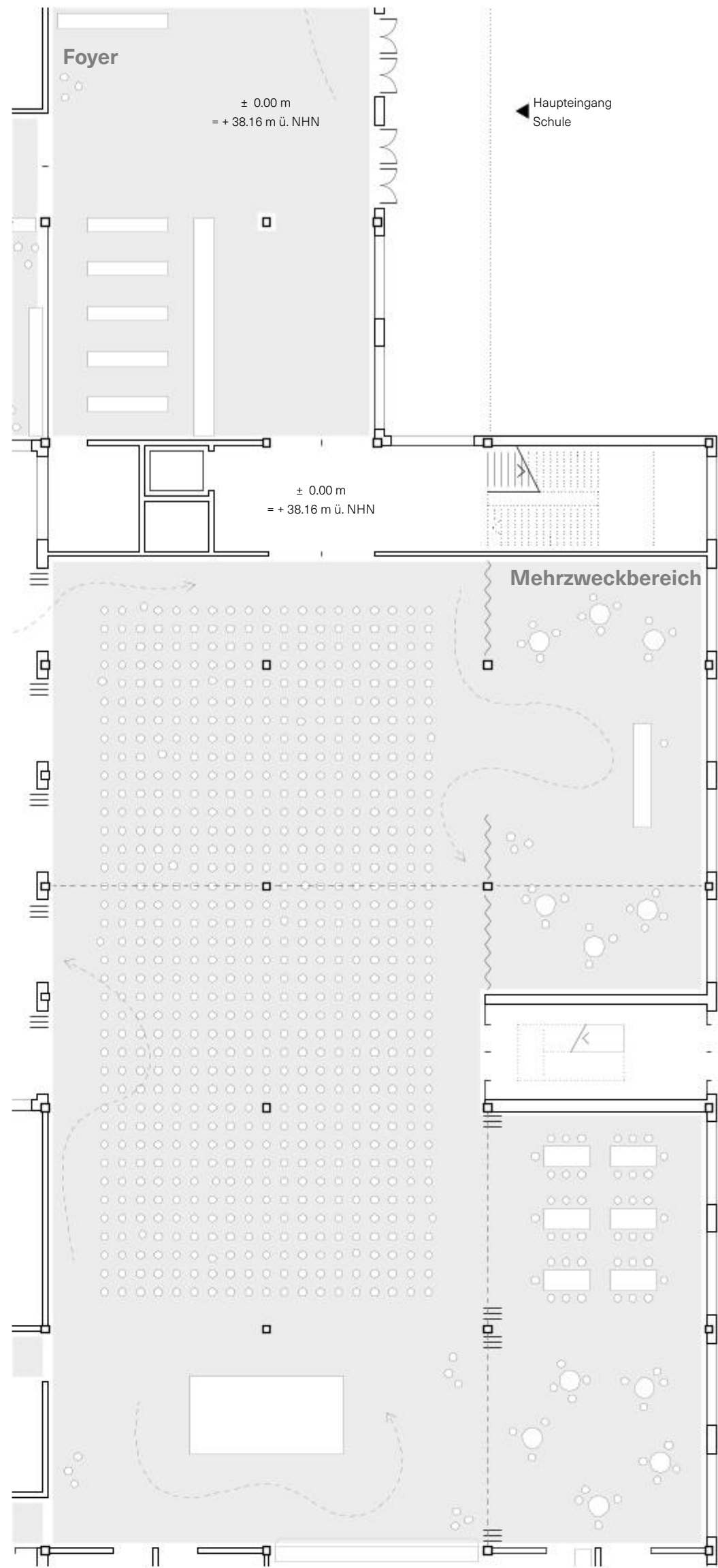
Grundrissausschnitt Erdgeschoss Mehrzweckbereich 1200
