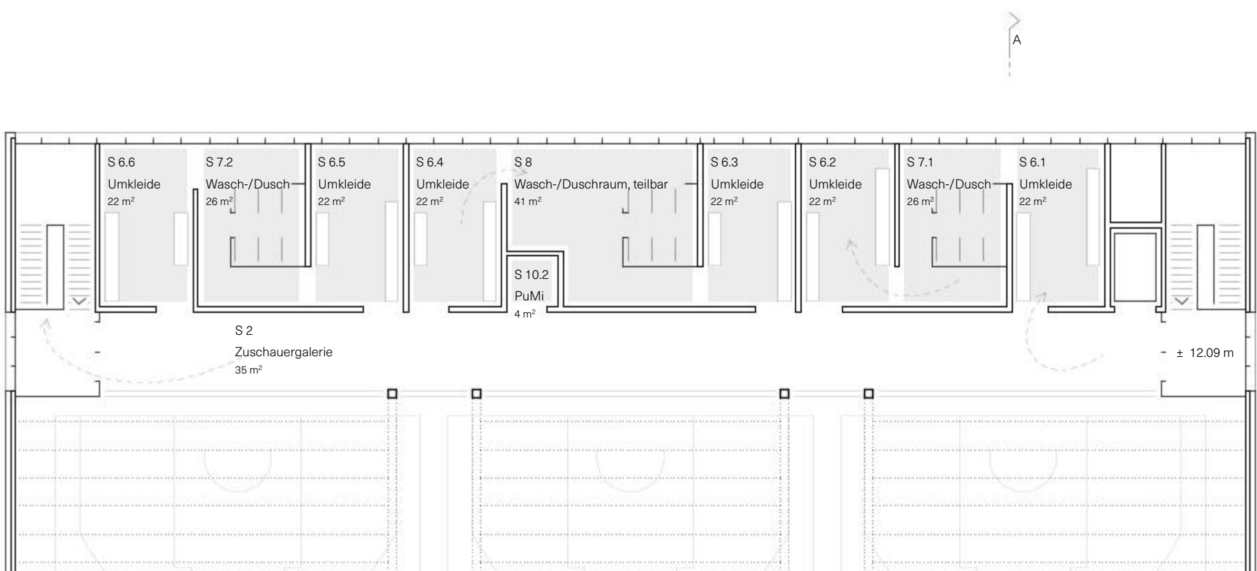
Grundrissausschnitt 3.Obergeschoss 1200
