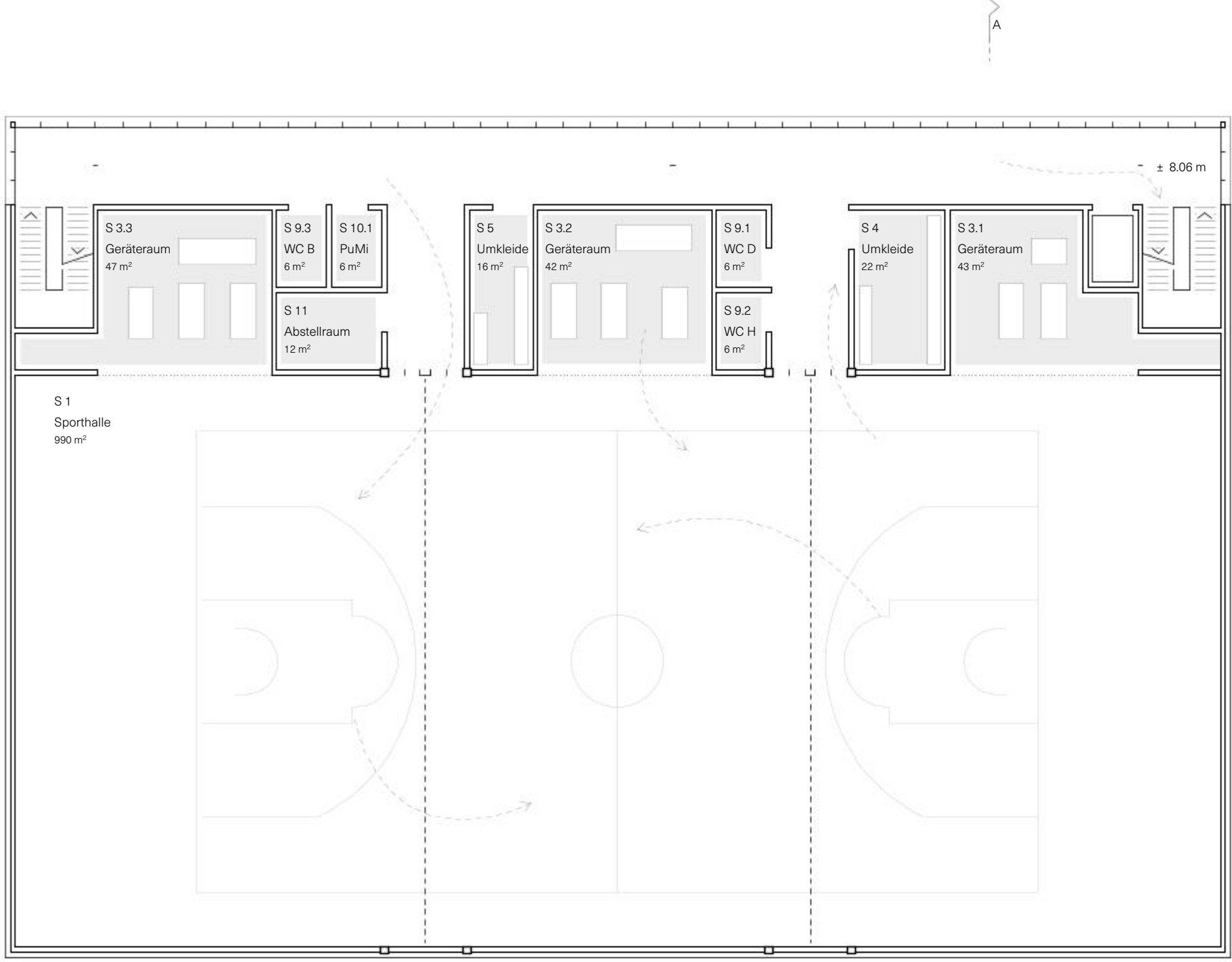
Grundrissausschnitt 3.Obergeschoss 1200
