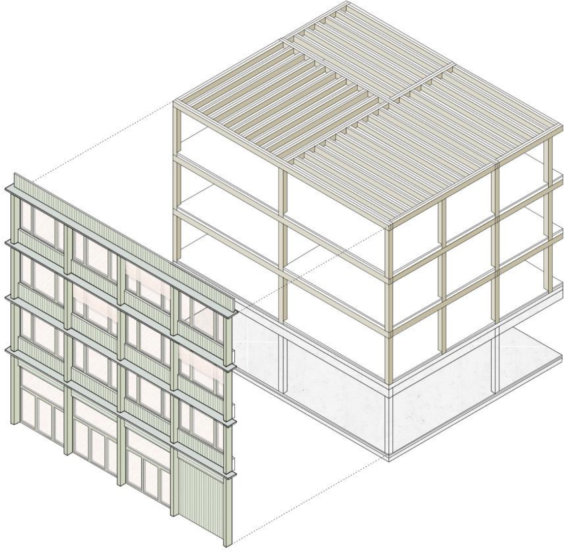
ELEMENTIERTE HOLZBAU - HOHER VORFERTIGUNGSGRAD
