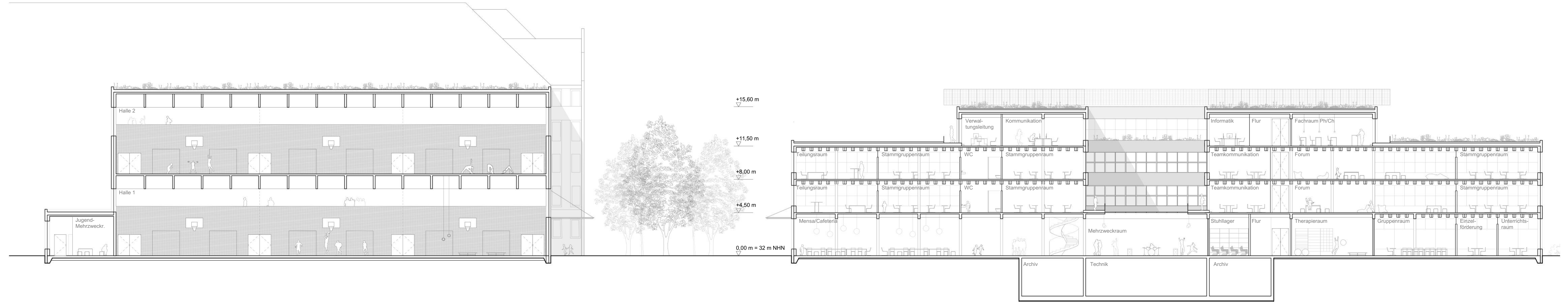
Querschnitt 1:200
