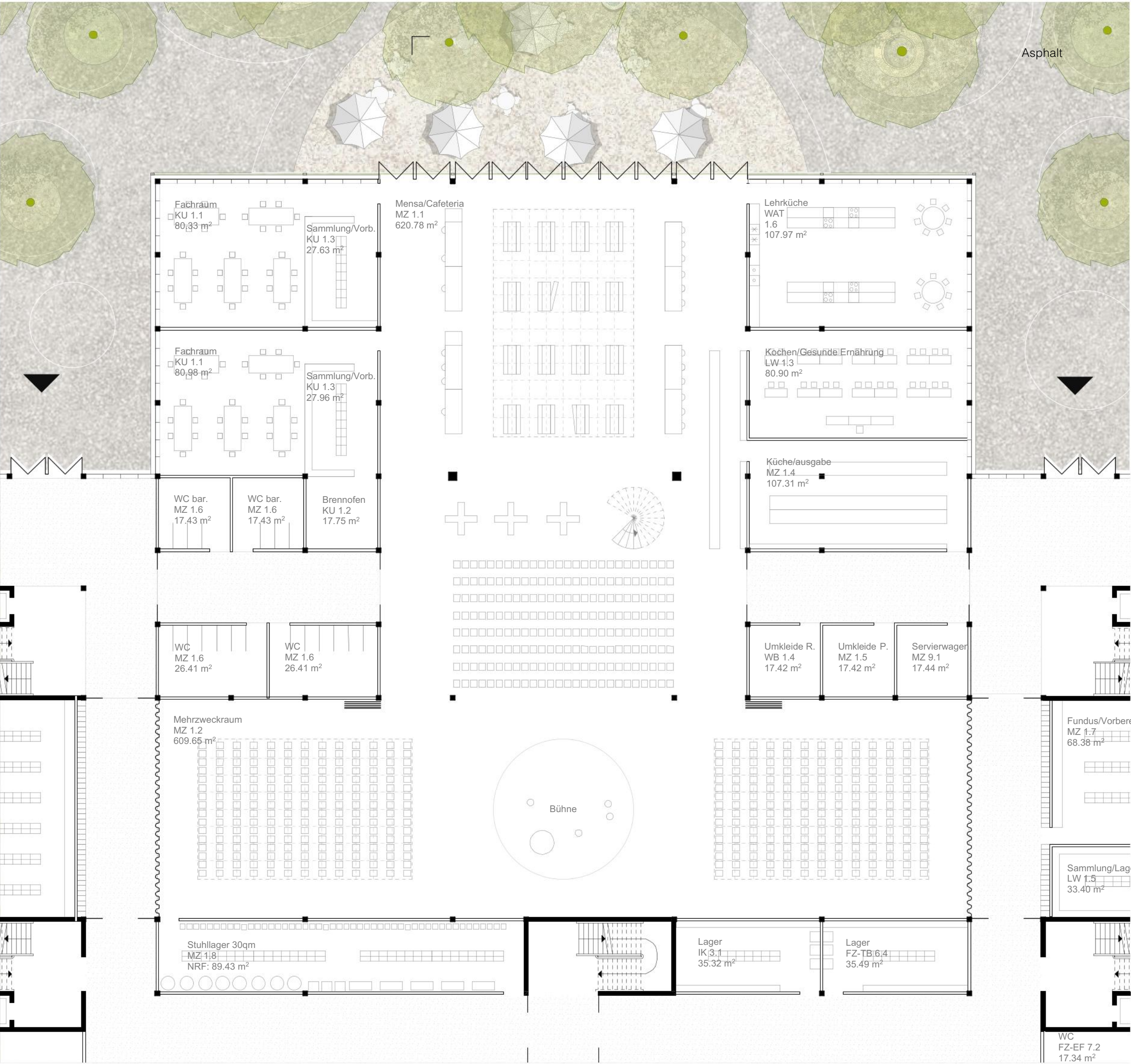
Grundrissausschnitt Mehrzweckbereich Veranstaltung 1:200
