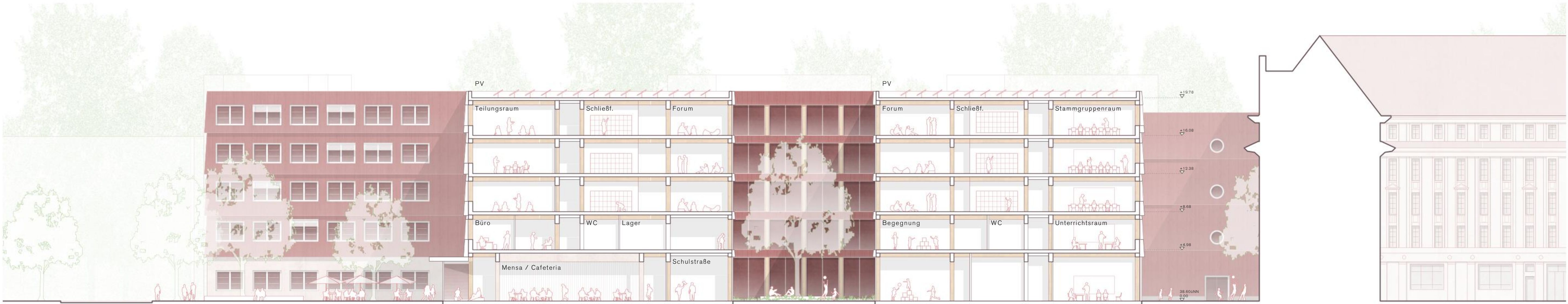
QUERSCHNITT 1.200
