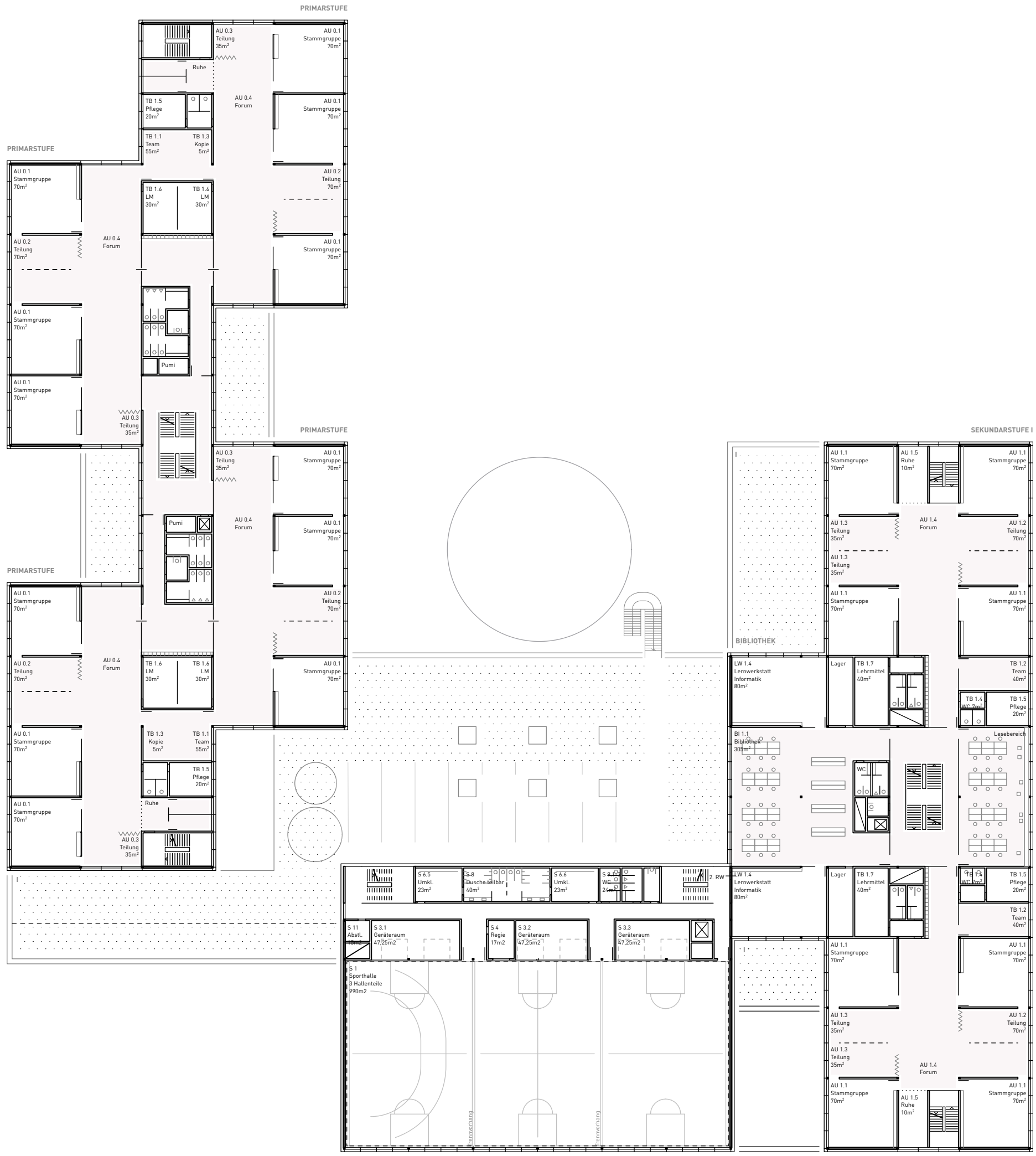
Grundriss 2. Obergeschoss 1 | 500
