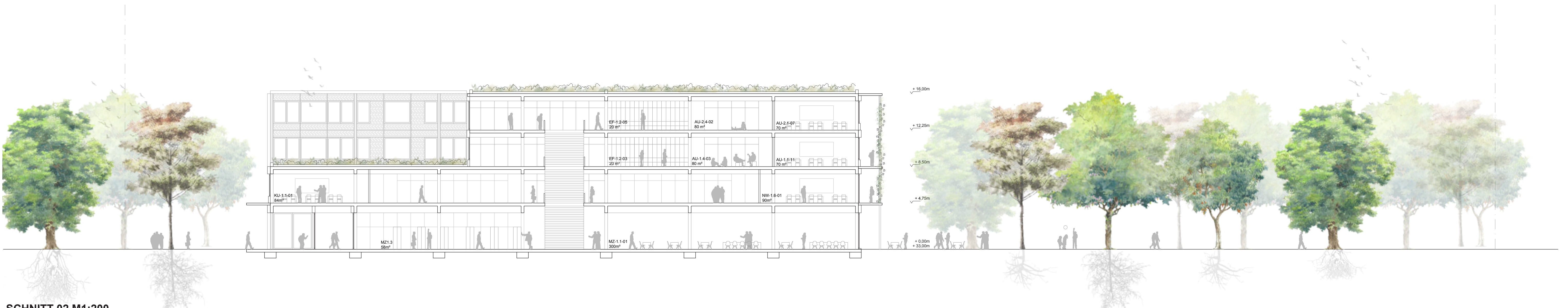
SCHNITT 02 M1:200
