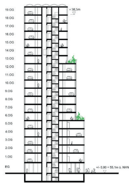
Schnitt Turm Typ A
