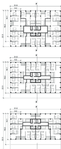
Regelgrundrisse Turm Typ A
