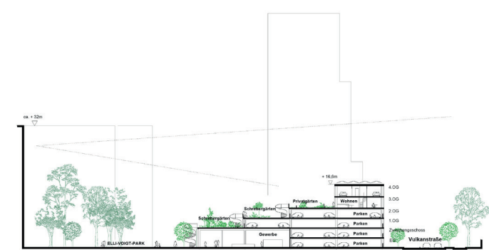
Schemaschnitt Terrassenhaus 1
