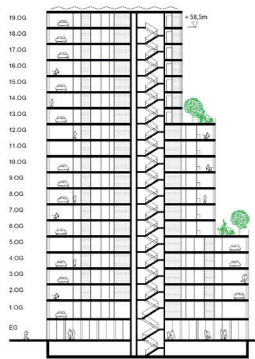
Schnitt Turm Typ B, 1:500
