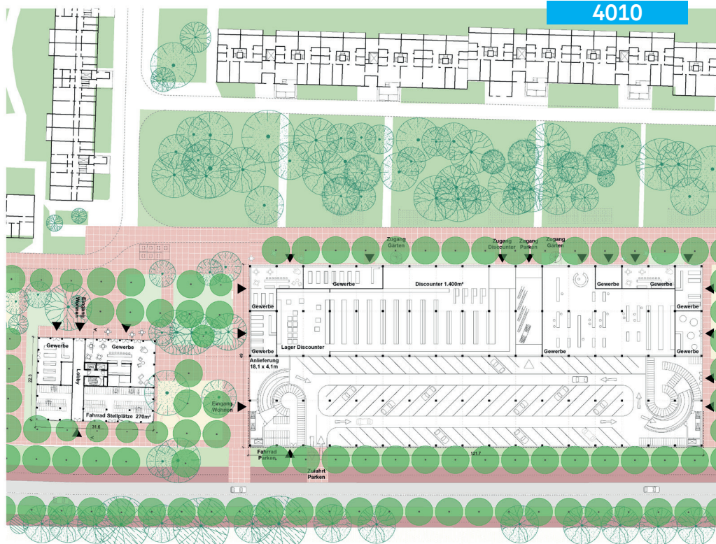
Edgeschoss Grundriss
