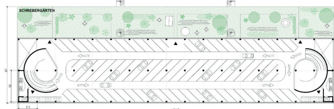
Grundriss 2.OG, Terrassenhaus 1
