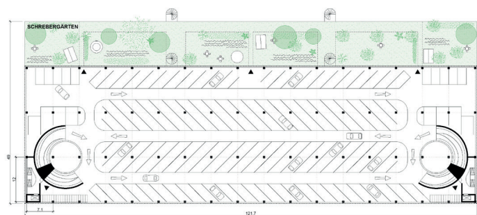
Grundriss 1.OG, Terrassenhaus 1
