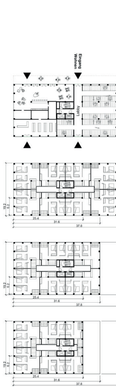
Regelgrundrisse Turm Typ B
