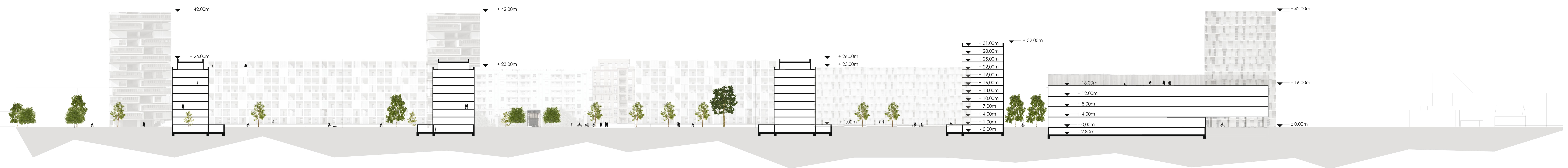
Schnitt Nord- Süd 1:500
