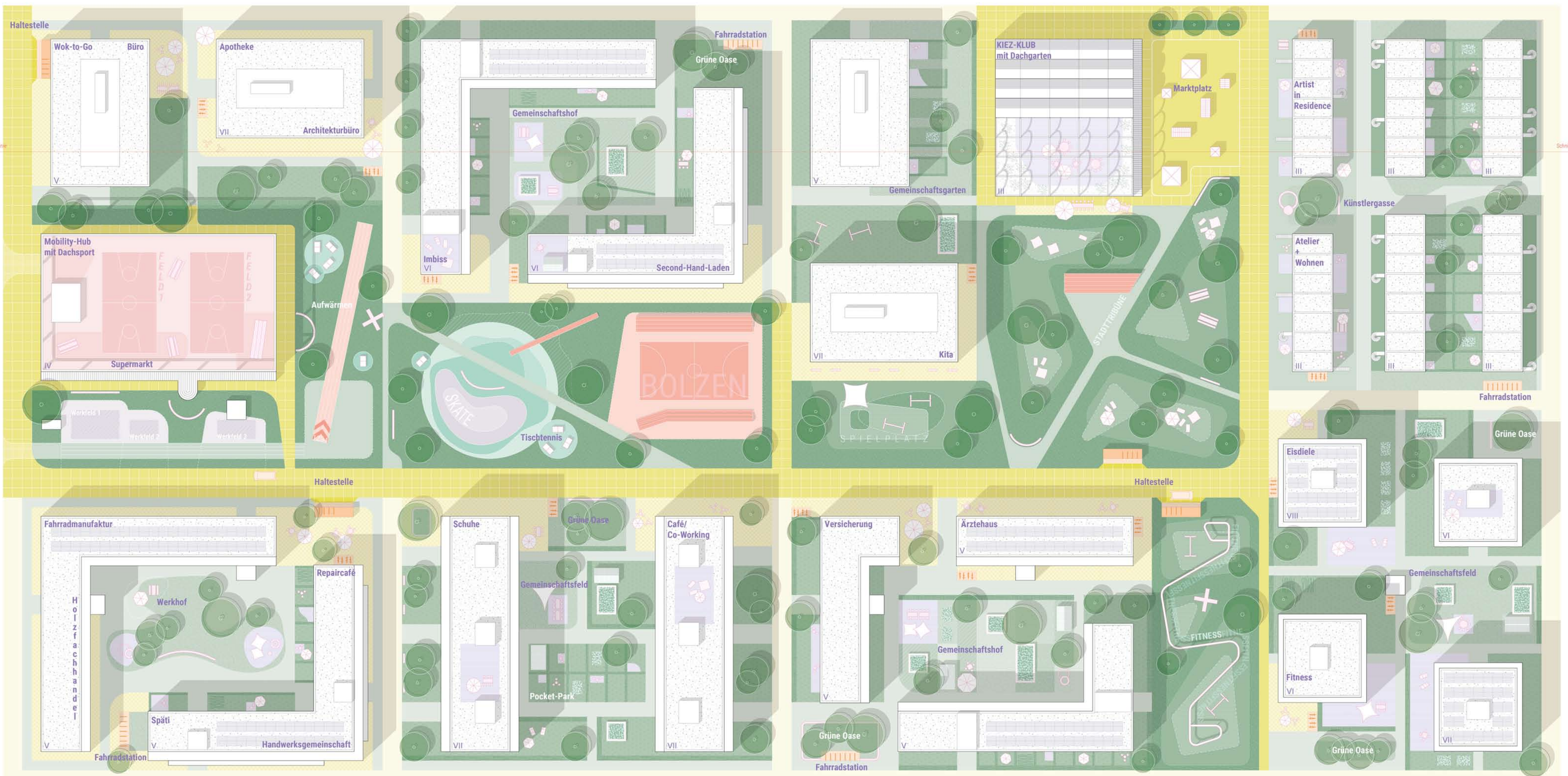
Lageplanausschnitt 1:500
